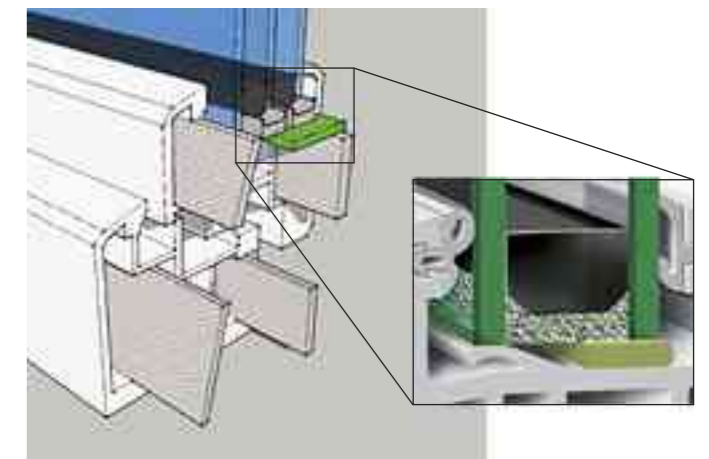
Bei der Produktion setzen Hochleistungsklebedüsen neue Maßstäbe für eine kraftschlüssige Verbindung.
