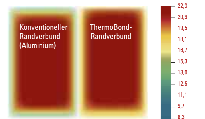
Infrarotaufnahme: Wärmebrücke im Vergleich
