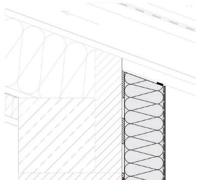
Abb. 28: Dachanschluss Warmdach
