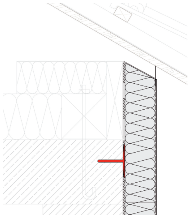
Abb. 29: Dachanschluss Kaltdach
