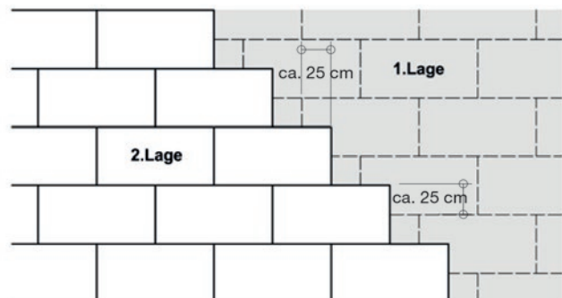
Abb. B.5: Verlegung der Dämmplatten / Verlegeraster
