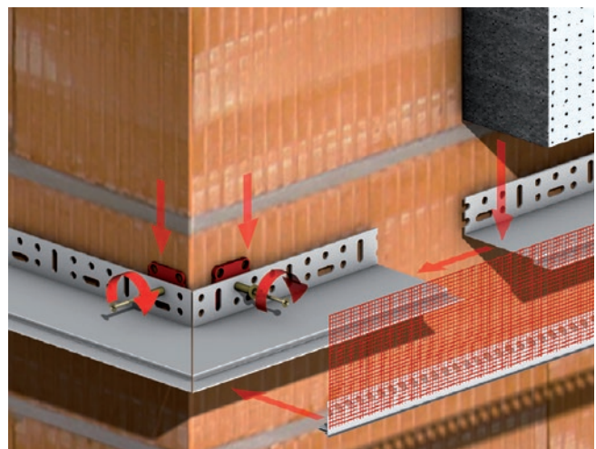
Abb. B.1: Baunit SockelProfil therm inkl. Tropfkante mit aufgeschweißtem Gewebe und Sockelprofil Montageset
