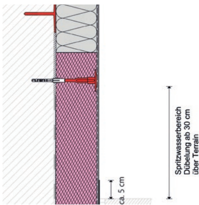
Abb. 8: Ebenflächiger Sockel
