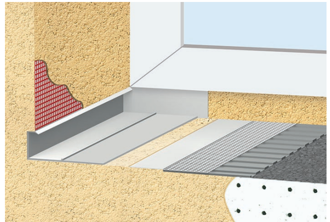
Abb. 27: Baumit FensterbankProfil
