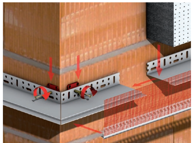
Abb. 10: Baunit SockelProfil therm
