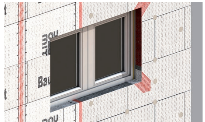
Abb. 31: Ausbildung der Bewehrung der Laibungen
