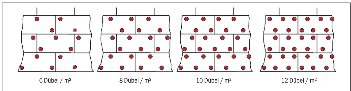
Abb. 24: W-Schema, bei Plattengröße \leq 0,5 \text{ m}^2
