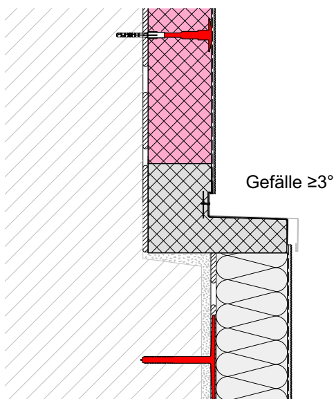
Abb. 9: Ausführung mit Baunit SohlbankanschlussProfil
