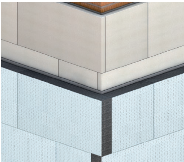
Abb. B.6: Verzahnte Ecksbildung
