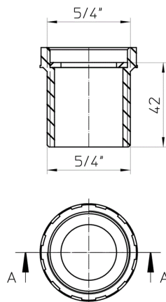
Schnitt A-A
