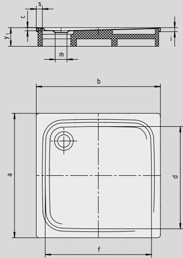
Modèle représenté : 400 avec support
