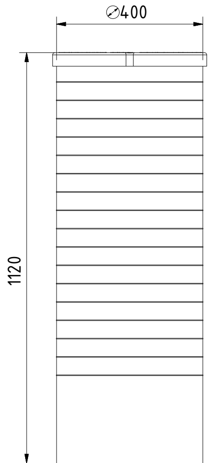
Ansicht von rechts vue de droit
