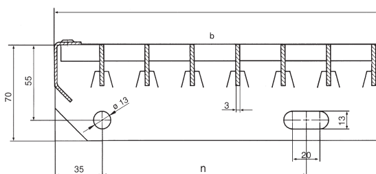
Seitenansicht: Stahlstufenrost Bohrmaße nach DIN 24531
