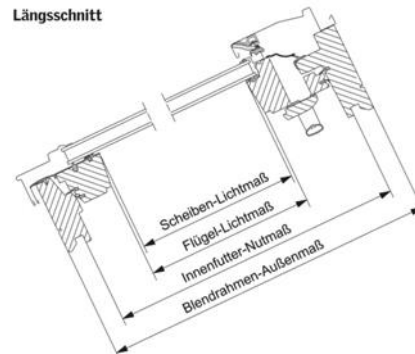
Längsschnitt
