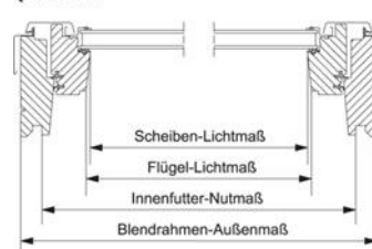
Längsschnitt
