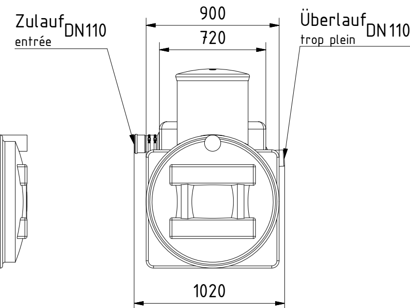
Ansicht von hinten vue de derrière
