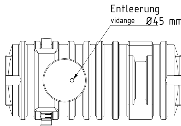
Ansicht von oben vue du dessus
