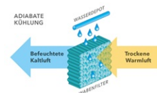
Luftkühler Funktionsprinzip
