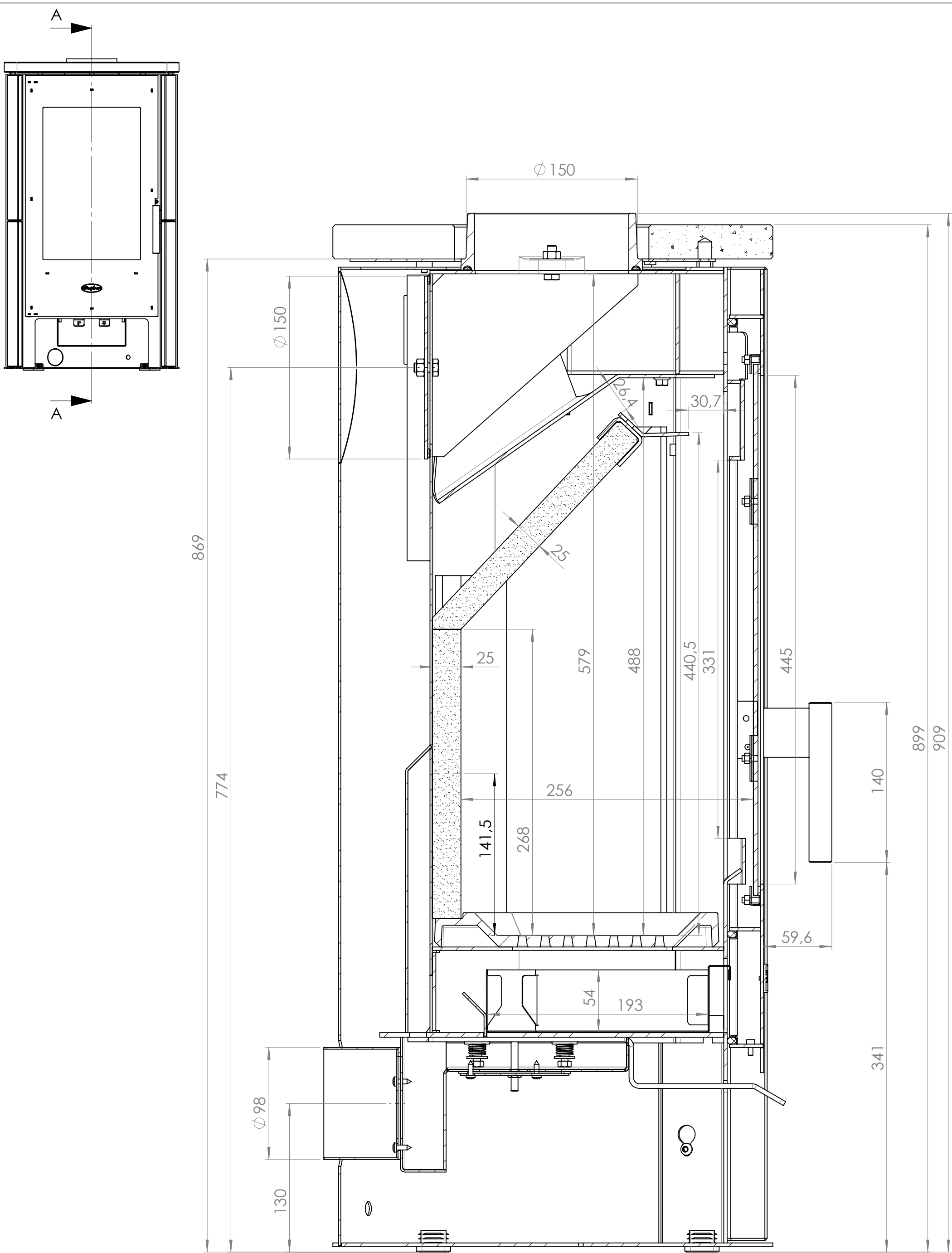
SECTION A-A SCALE 1 : 3
