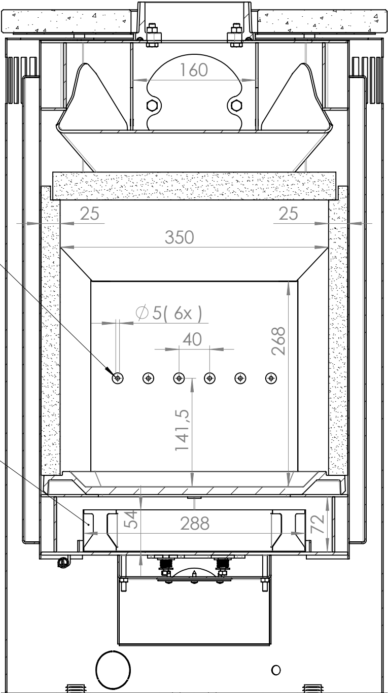
SECTION D-D SCALE 1 : 5
