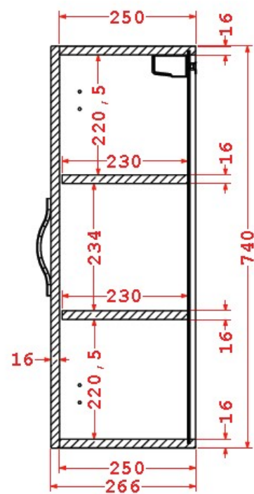
SEZIONE A-A
