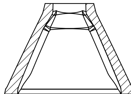
SEZIONE A-A
