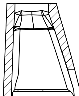
SEZIONE B-B
