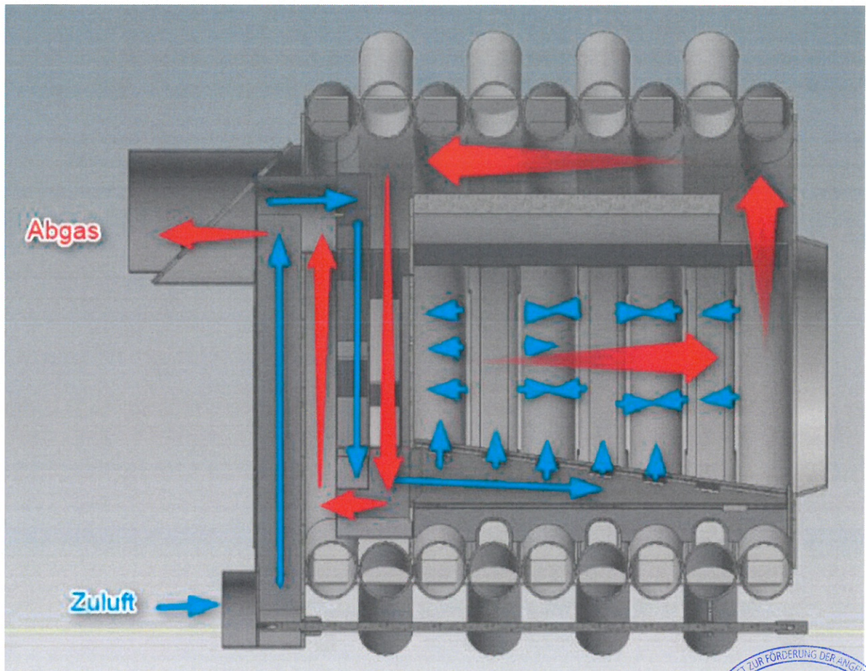
Luft- und Abgaswege im Raumheizer » Kanuk 00 – 7 kW «
