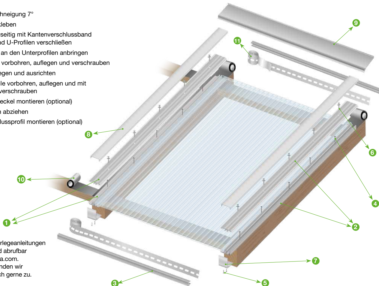
Mittelpprofil 16 mm Art.-Nr.: 3441163 ff
