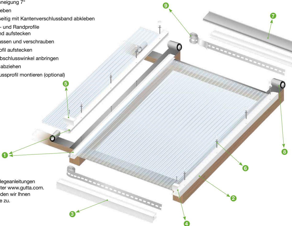
1 Mittelprofil 10 oder 16 mm Art.-Nr.: 3442123 ff
