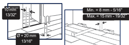
DEHNUNGSFUGE
