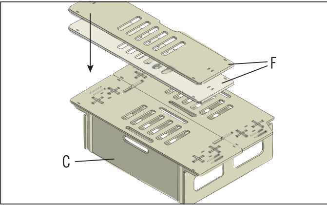
Zum Montieren der beiden weiteren Abdeckplatten (F) die Frontplatte (C) nach vorne herausziehen.
