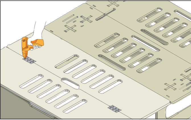
Richte die Platten so aus, dass die Grifföffnung zwischen beiden Platten ist. Verbinde sie mit zwei Scharnieren und Schrauben von 3x16 mm.
