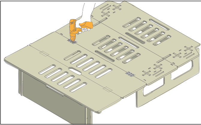
Die beiden Platten umdrehen und an den zuvor aufgesteckten Abdeckplatten mit zwei Scharnieren und Schrauben von 3x16 mm anschrauben. Ausgezogen bietet das Bett eine max. Liegefläche von L: 1800 mm x B: 1500 mm x H: 415 mm und zusammengeschoben eine Fläche von L: 1000 mm x B: 1500 mm x H: 415 mm.
