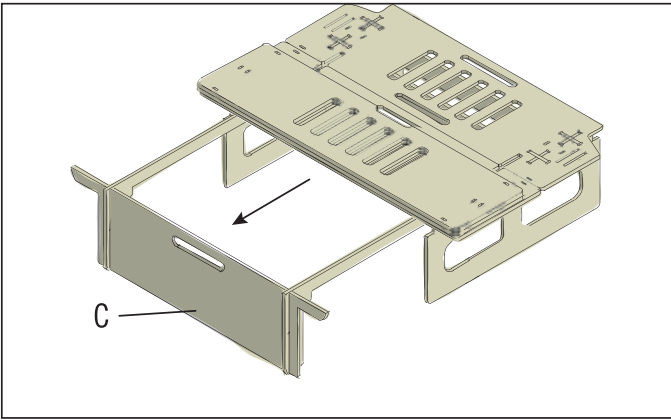
Lege die Abdeckplatten mit der Rückseite nach oben auf das herausgezogene Bauteil.
