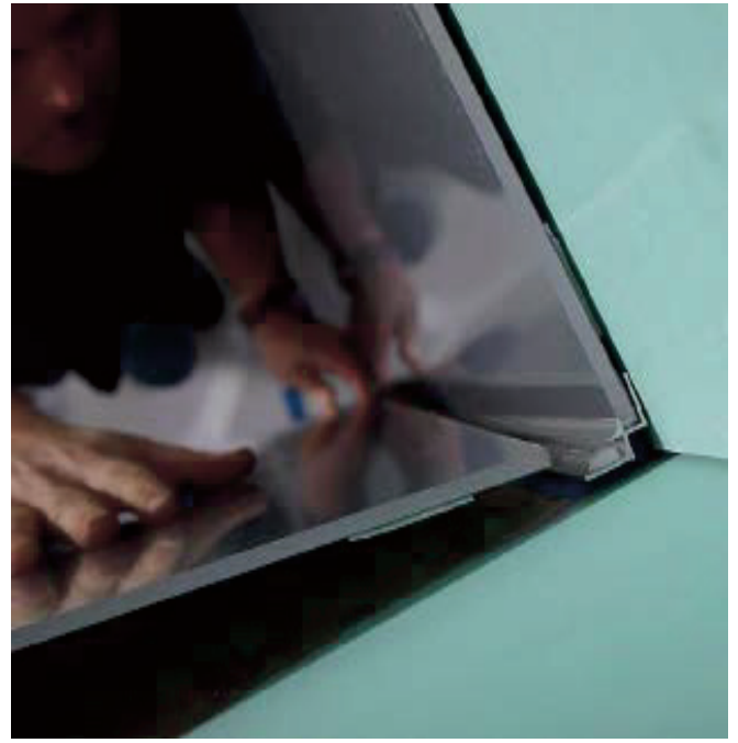
3.18 Beim Setzen der zweiten Platte wieder aus der Ecke beginnend anlegen und andrücken.
