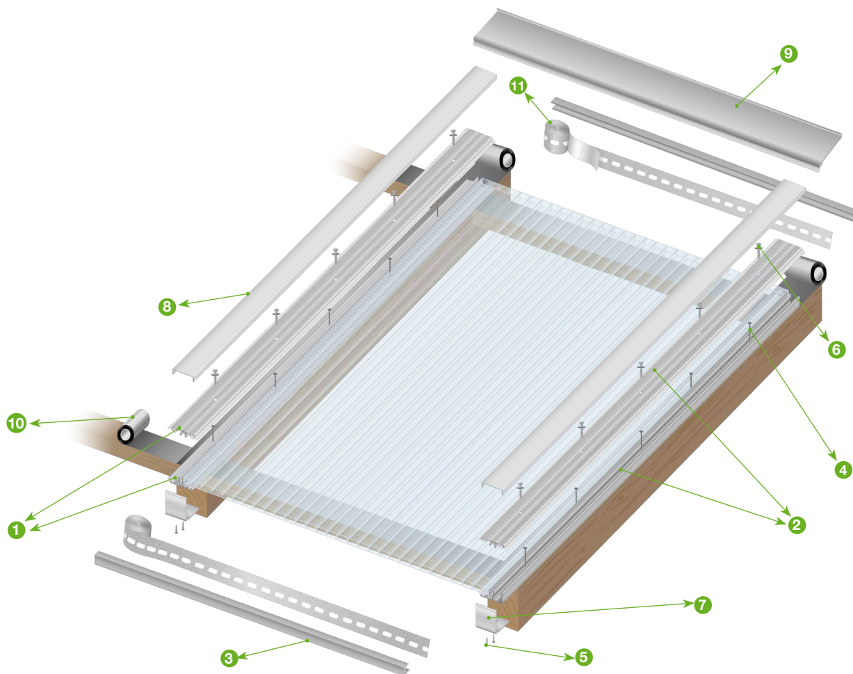
Mittelprofil 16 mm Art.-Nr.: 3441163 ff
