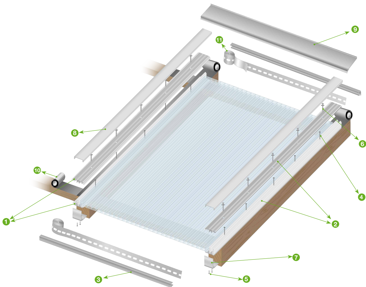
1 Mittelpfprofil 25 mm Art.-Nr.: 3441163 ff
