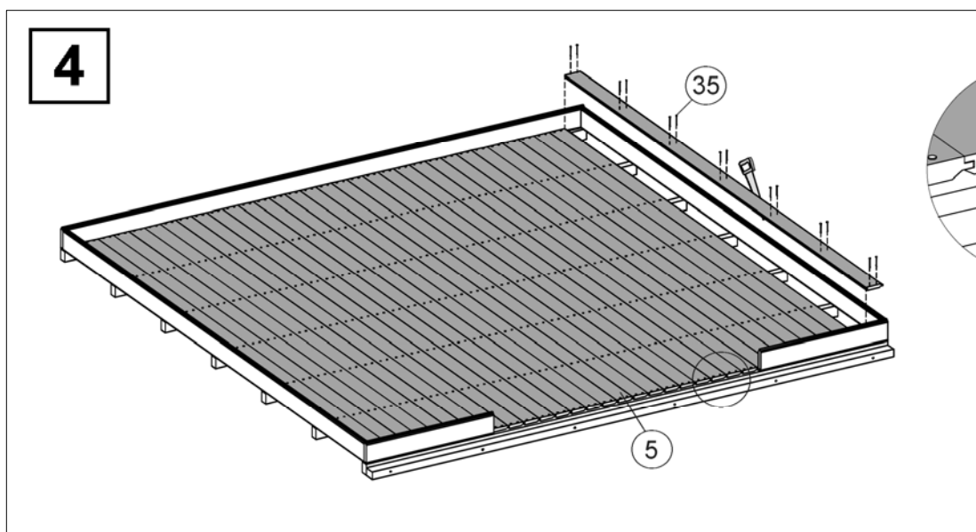
Abbildung Art.-Nr.: 225.3030
