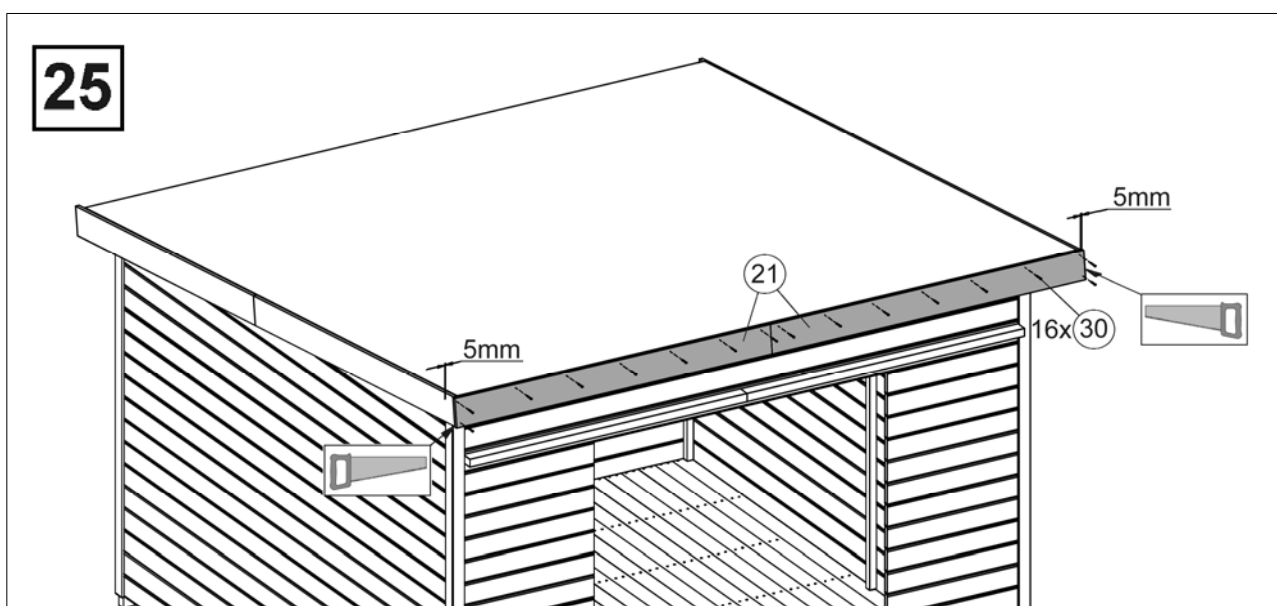
Abbildung Art.-Nr.: 225.3030
