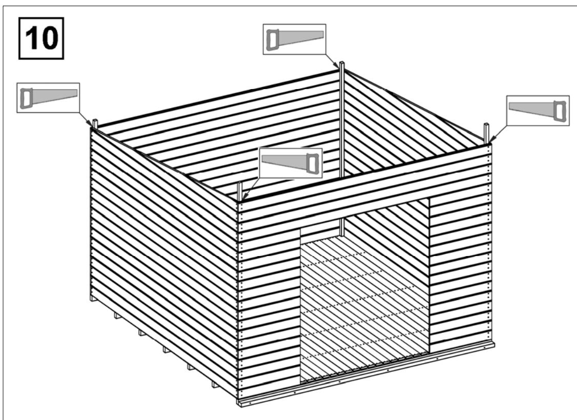
Abbildung Art.-Nr.: 225.3030
