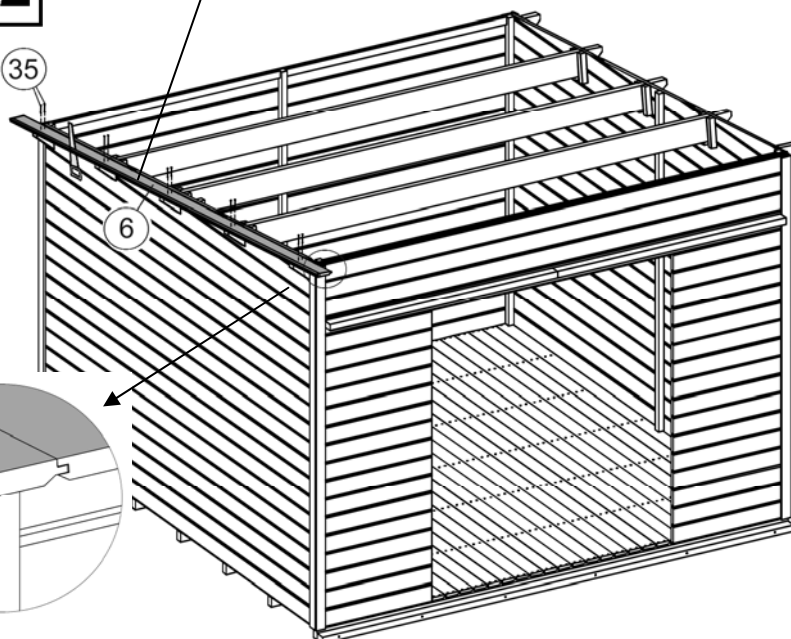
Abbildung Art.-Nr.: 225.3030
