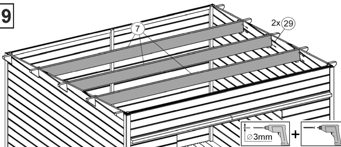
Abbildung Art.-Nr.: 225.3030
