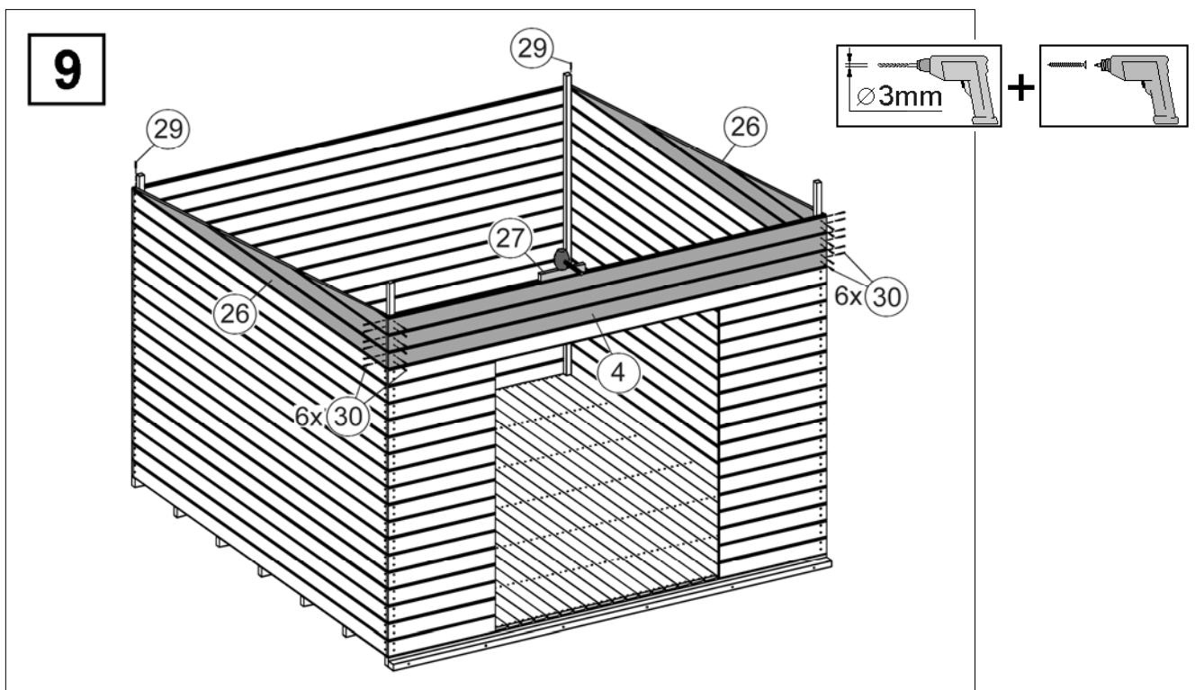
Abbildung Art.-Nr.: 225.3030
