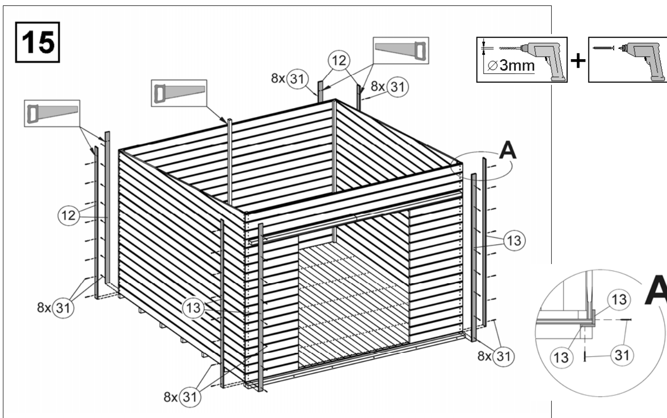
Abbildung Art.-Nr.: 225.3030
