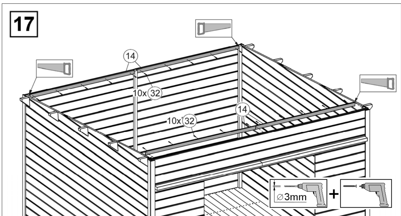
Abbildung Art.-Nr.: 225.3030
