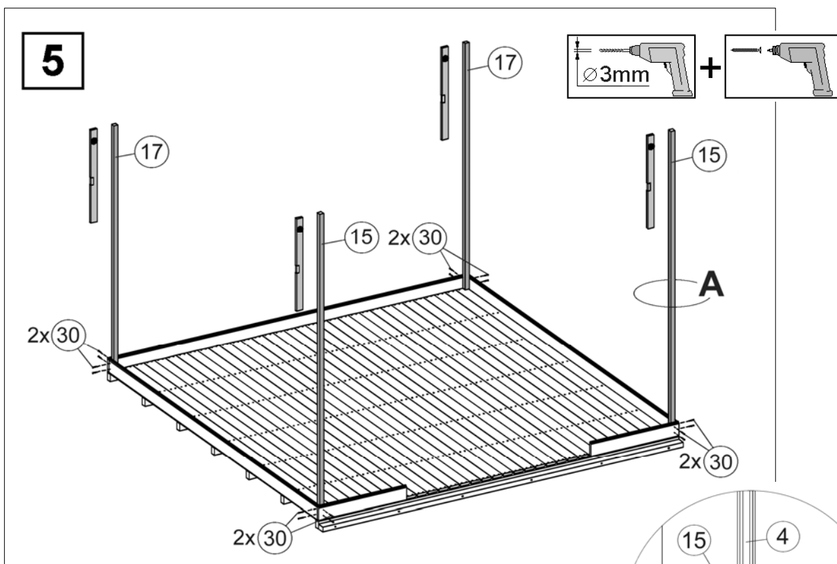
Abbildung Art.-Nr.: 225.3030
