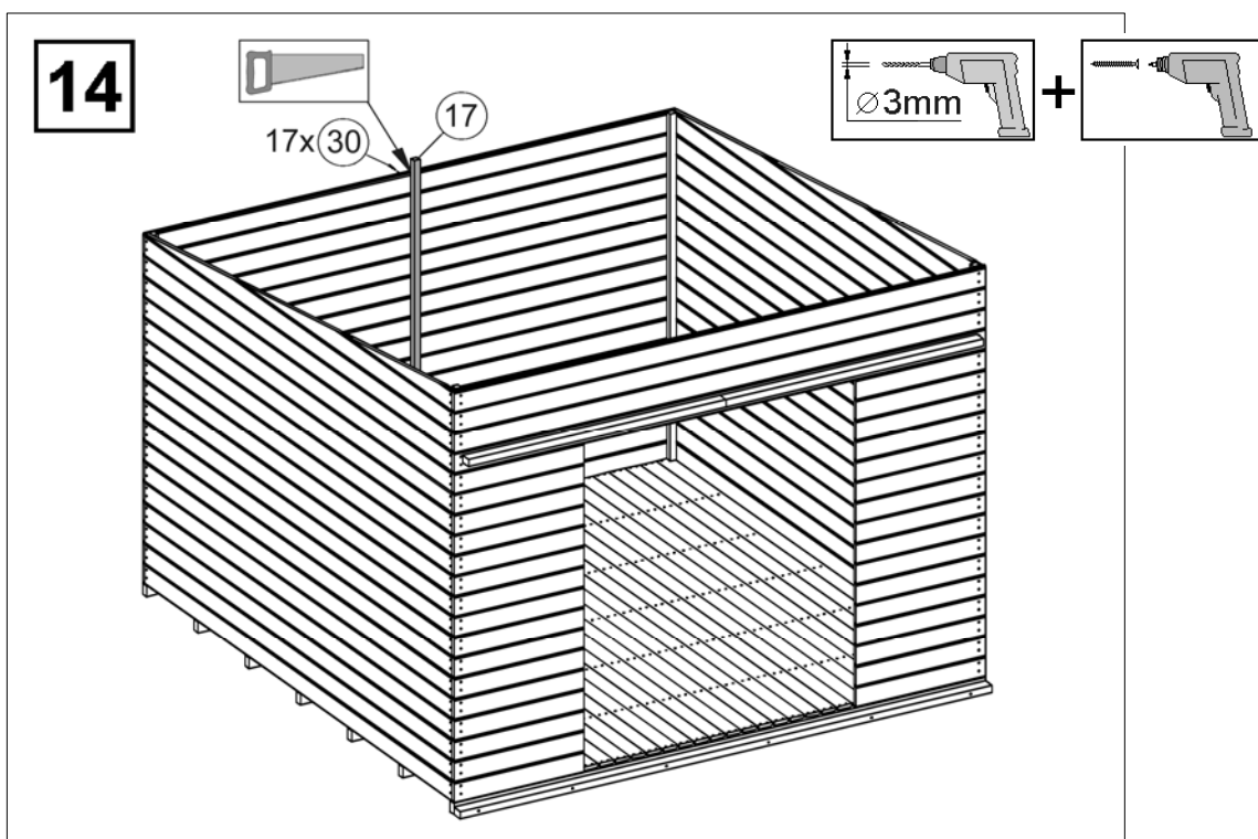
Abbildung Art.-Nr.: 225.3030
