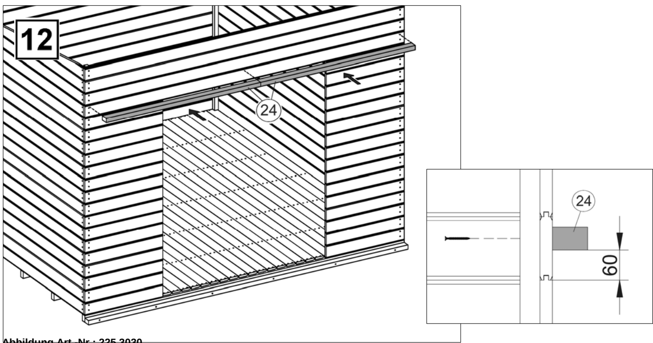
Abbildung Art.-Nr.: 225.3030
