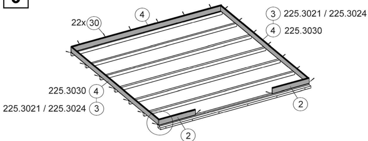
Abbildung Art.-Nr.: 225.3030
