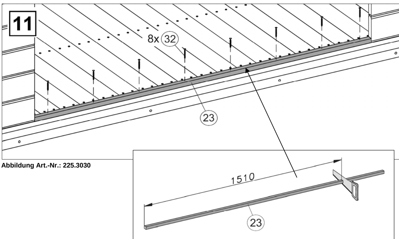
Abbildung Art.-Nr.: 225.3030
