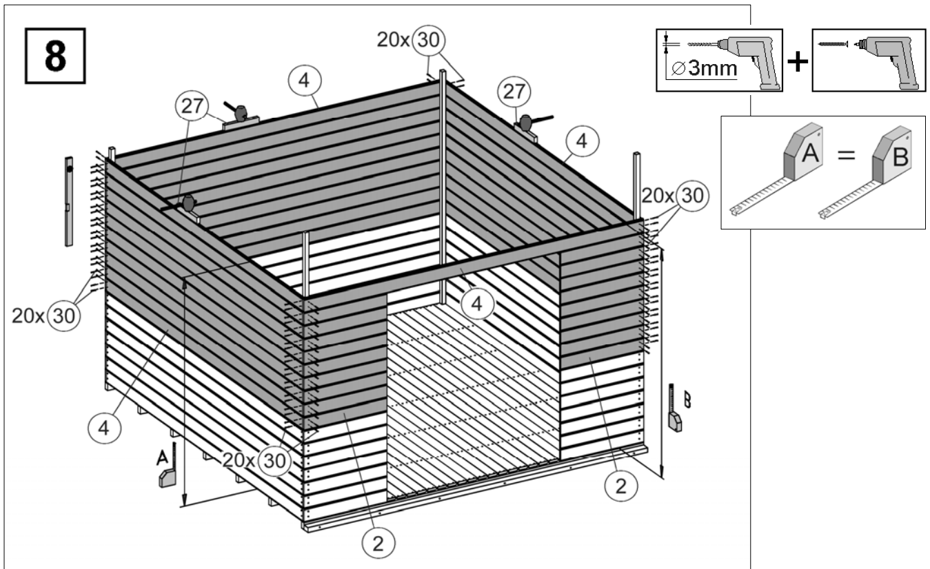
Abbildung Art.-Nr.: 225.3030
