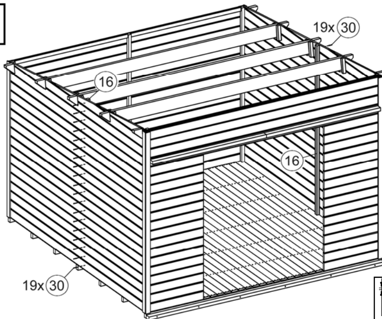
Abbildung Art.-Nr.: 225.3030
