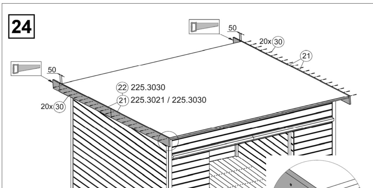
Abbildung Art.-Nr.: 225.3030
