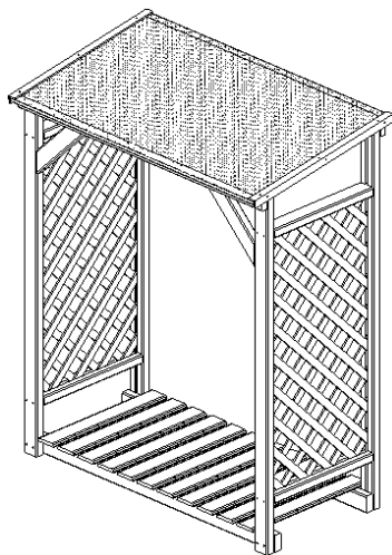
3) Artikel 355/03 Wetterschutz für Kaminholzregale
