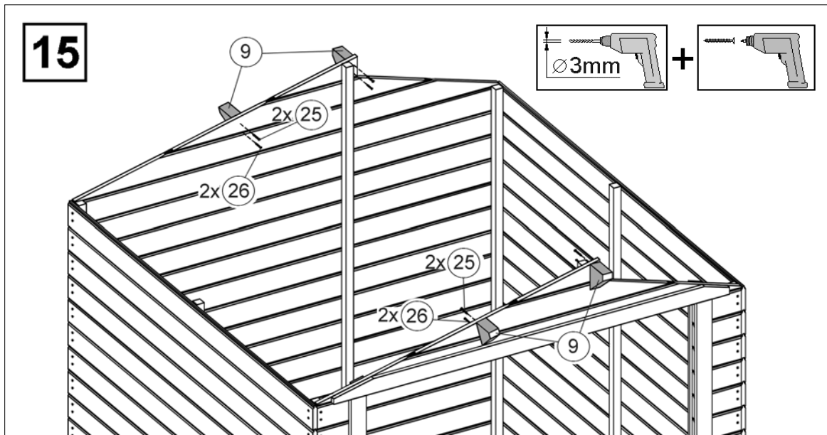
Abbildung Art.-Nr.: 323.2020
