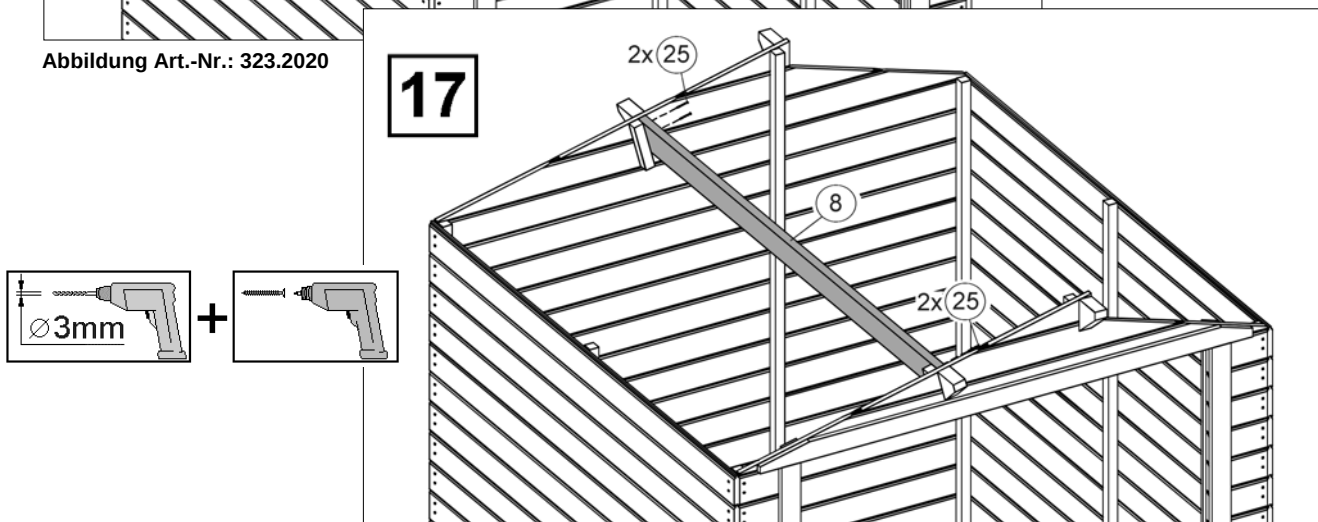
Abbildung Art.-Nr.: 323.2020
