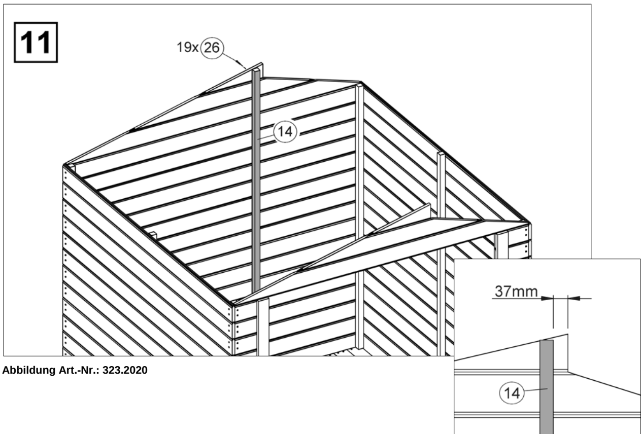
Abbildung Art.-Nr.: 323.2020
