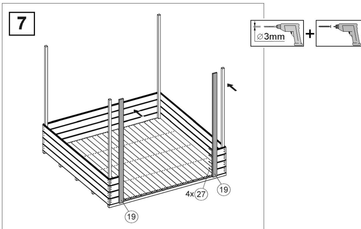
Abbildung Art.-Nr.: 323.2020
