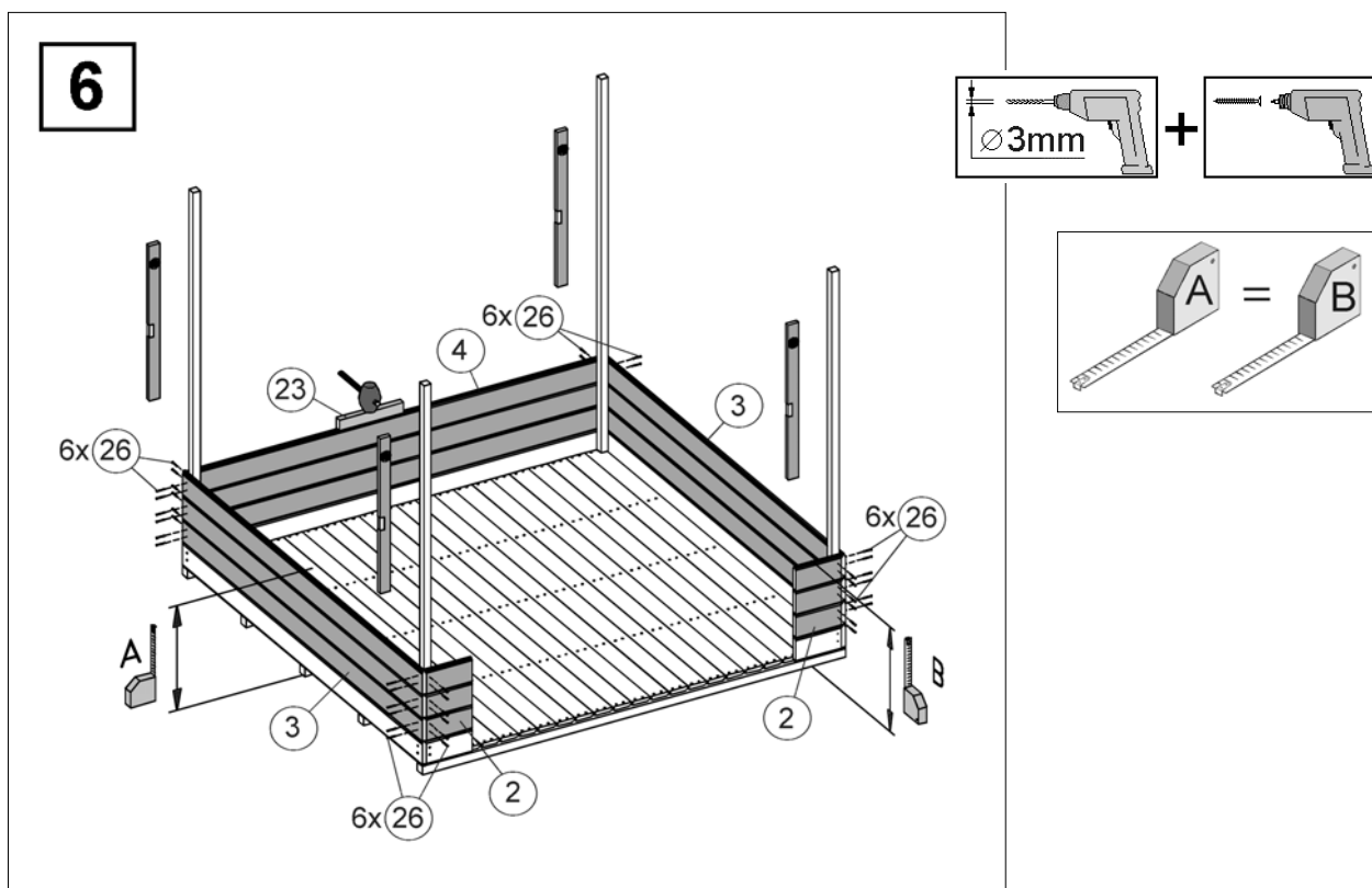
Abbildung Art.-Nr.: 323.2020
