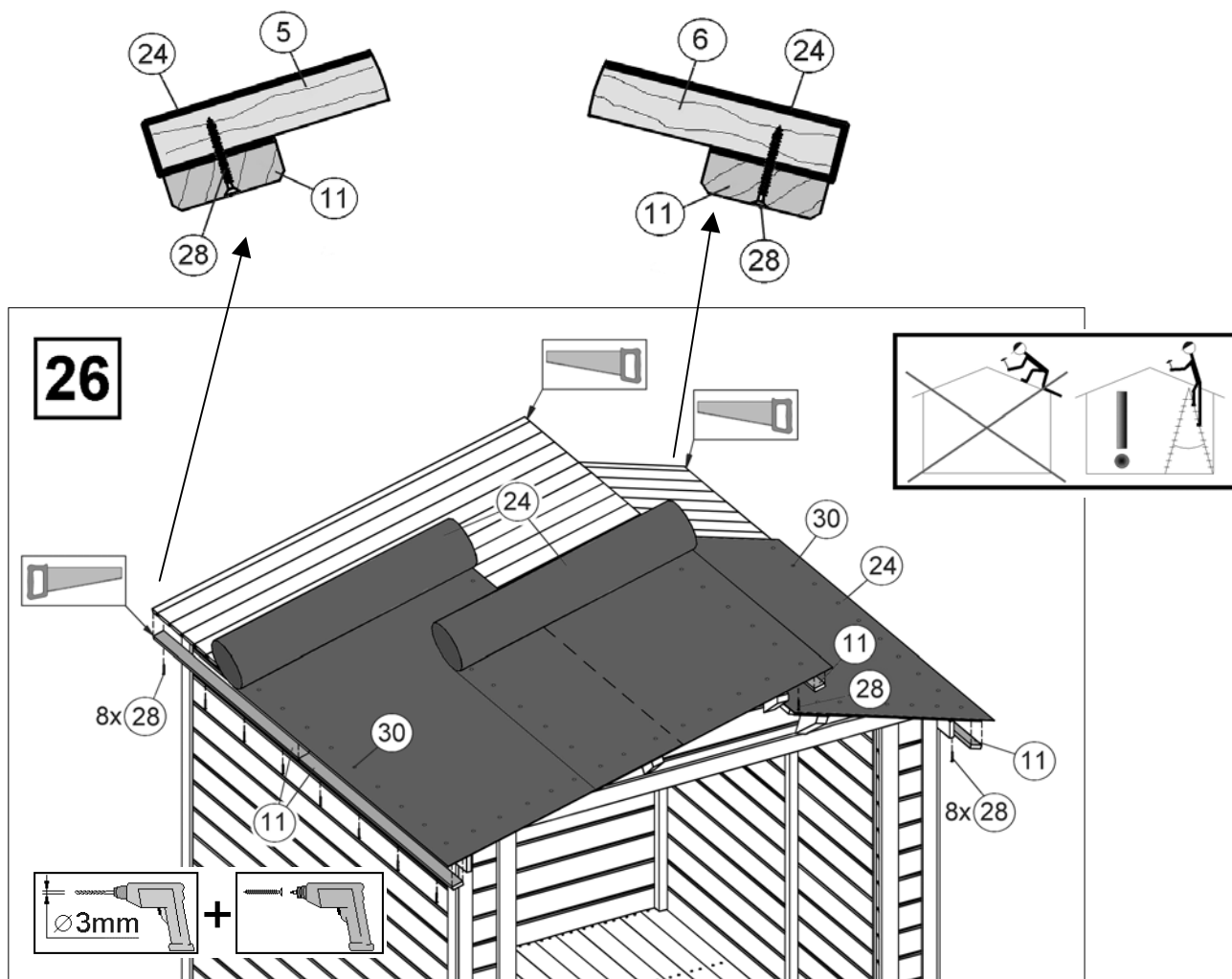
Abbildung Art.-Nr.: 323.2020
