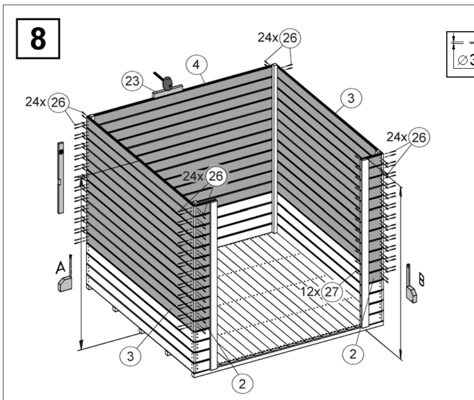
Abbildung Art.-Nr.: 323.2020
