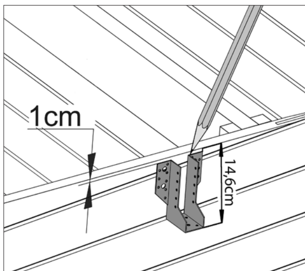
Abb. Art.-Nr.: 219.3030.40241
