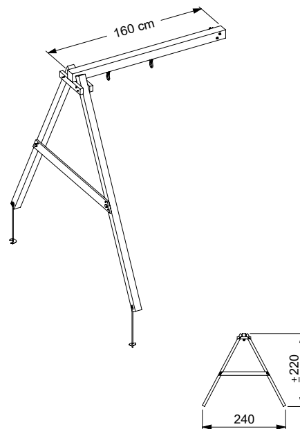
1-Swing Module 220
