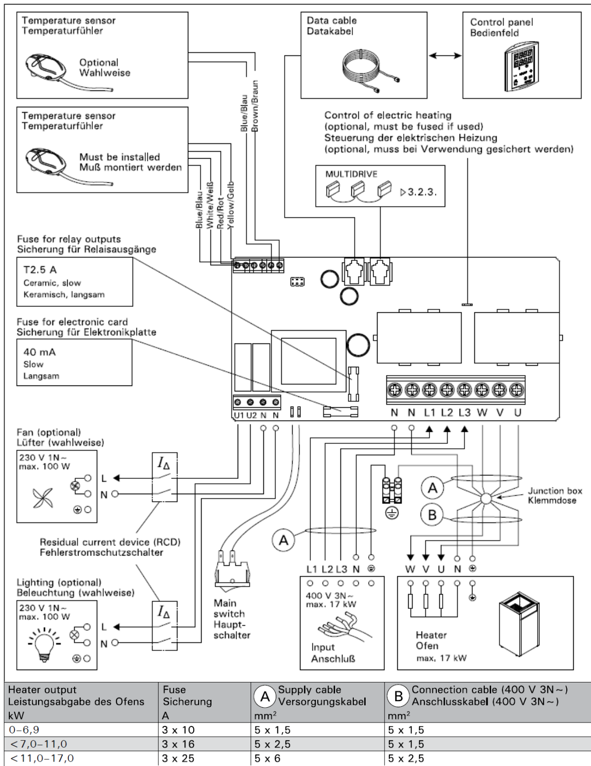
Abbildung 11. Elektroanschlüsse des Steuergerät und des Saunaofens
