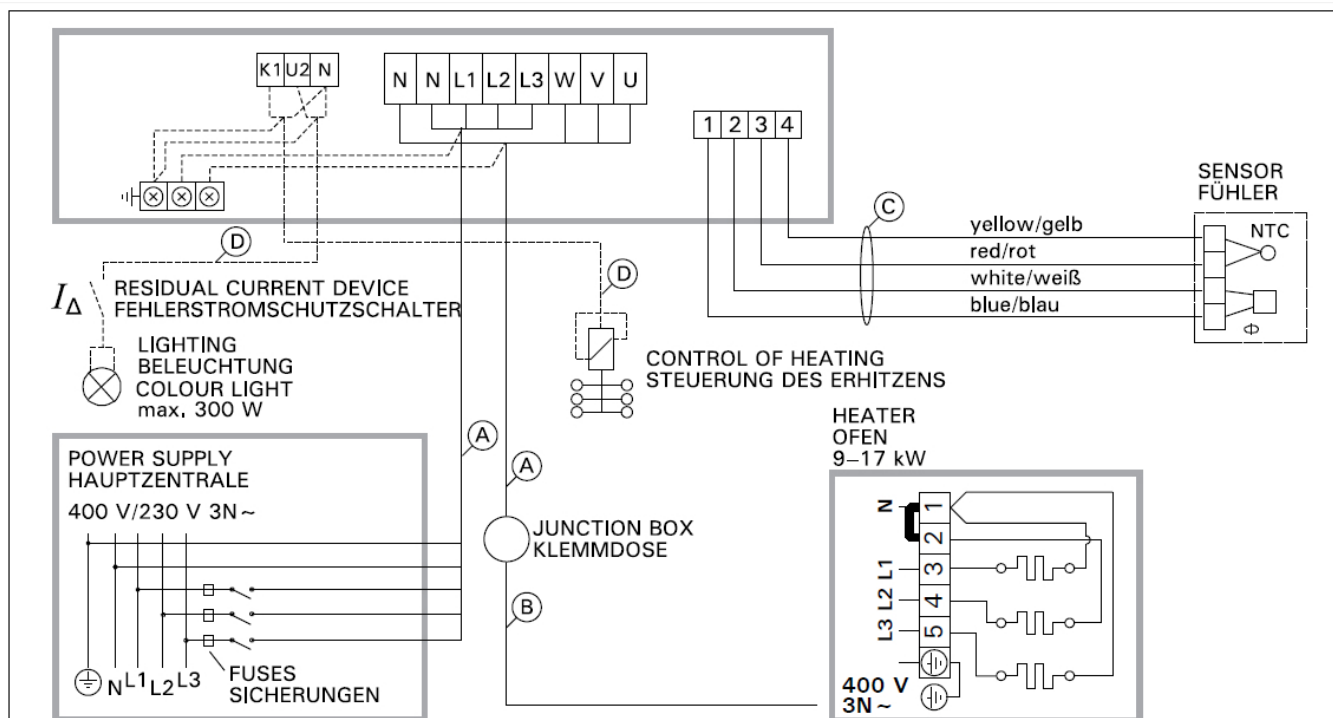
Abbildung 9. Elektroanschlüsse
