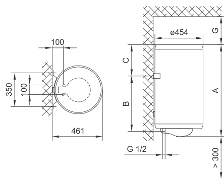
Dimensions du chauffe-eau pour le raccordement et le montage [mm]
