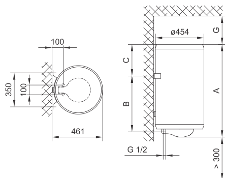
Anschluss- und Montagedimensionen des Warmwasserbereiters [mm]
