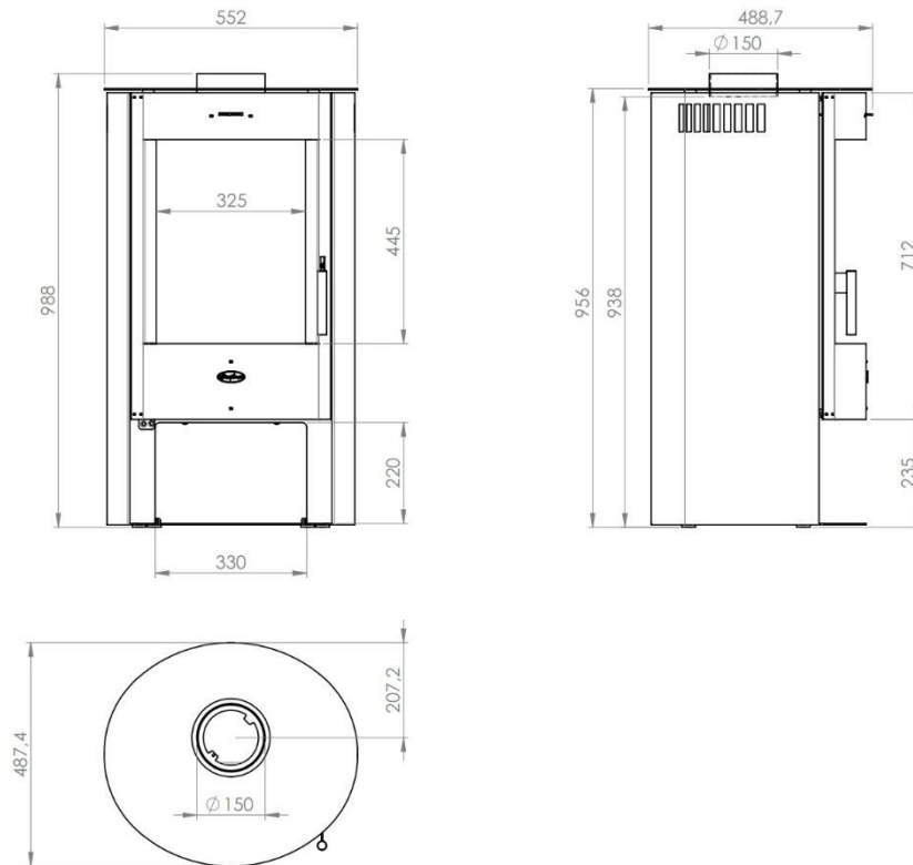
Abbildung 11 - Hauptmaße
