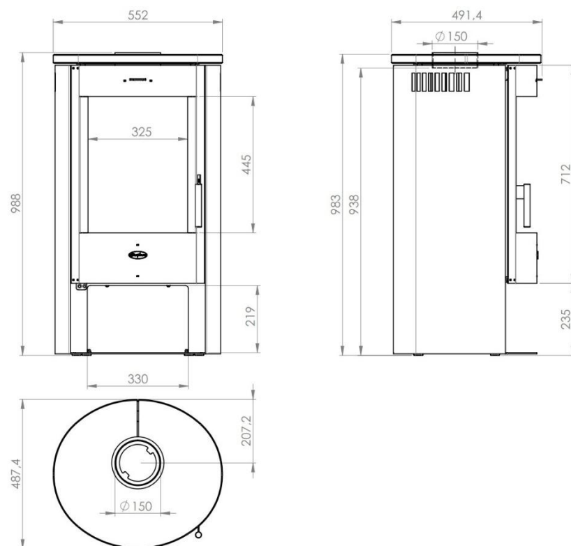
Abbildung 10 - Hauptmaße
