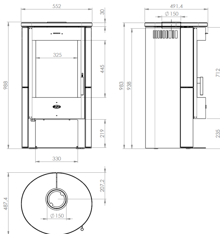
Abbildung 3 – Hauptmaße
