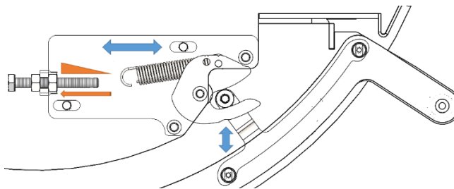
Abbildung 20 – Schnappverschluss (nur für Versionen: R5688/R5693)
