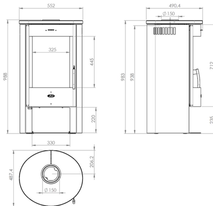
Abbildung 5 - Hauptmaße
