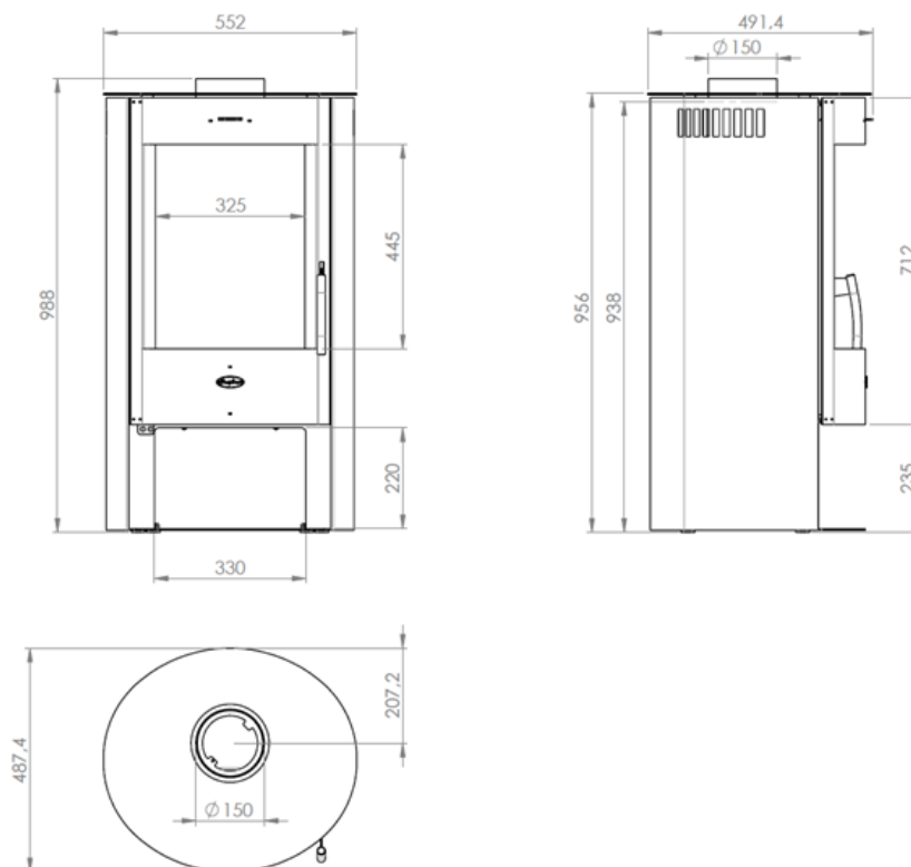
Abbildung 4 – Hauptmaße
