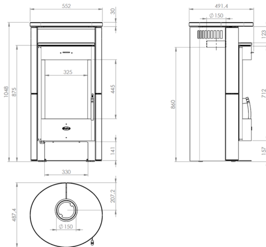
Abbildung 7 – Hauptmaße
