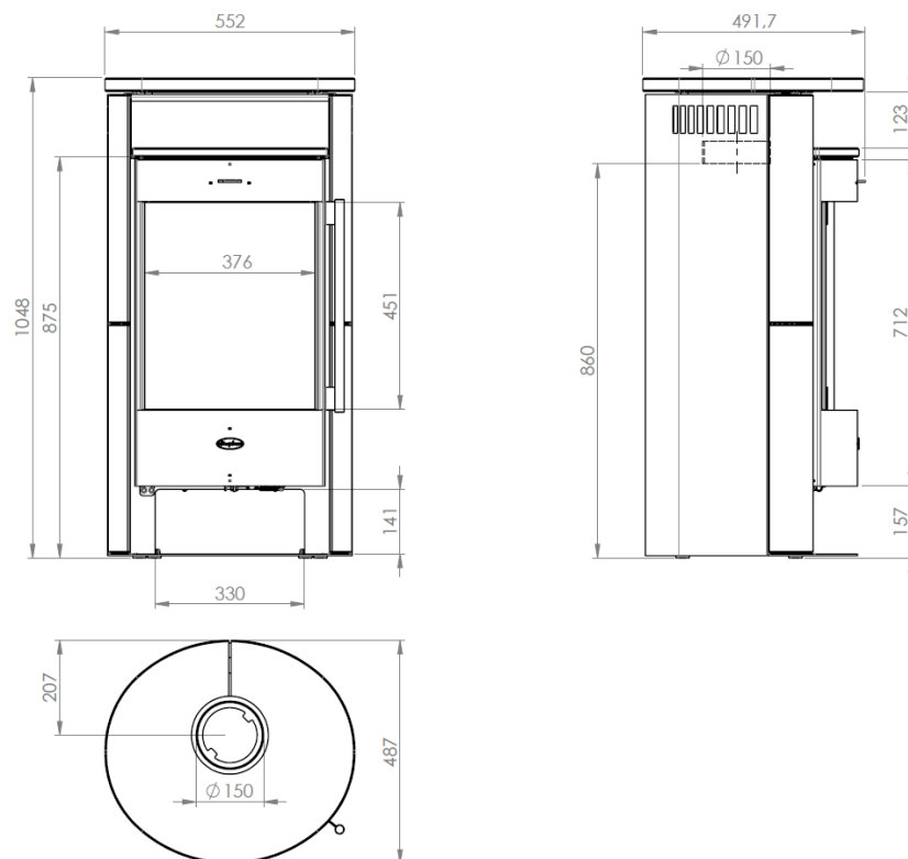
Abbildung 6 - Hauptmaße
