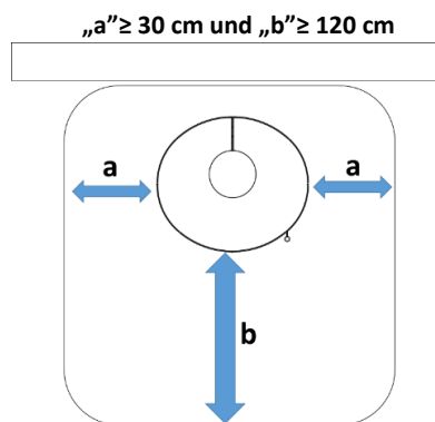
Abbildung 13 – Bodenplatte
