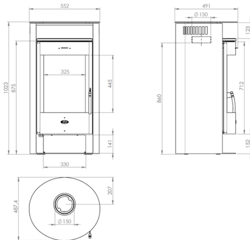
Abbildung 9 - Hauptmaße
