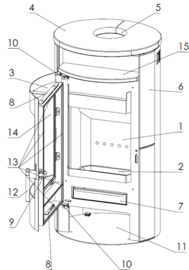
Abbildung 1 – Aufbau des Geräts
