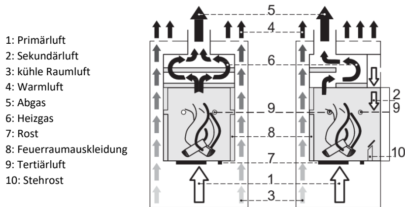
Abbildung 12 – Fire-Plus System, schematische Darstellung
