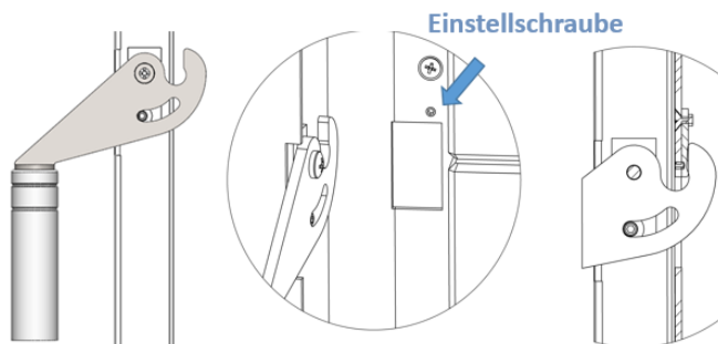
Abbildung 21 – Verriegelung der Tür
