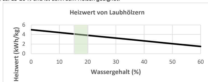
Abbildung 15 - Heizwertänderung in Abhängigkeit vom Wassergehalt
