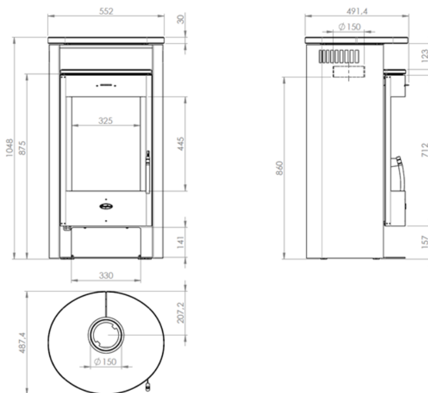
Abbildung 8 - Hauptmaße
