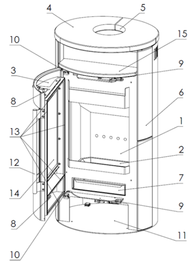
Abbildung 2 - Aufbau des Geräts /R5688 & R5693/
