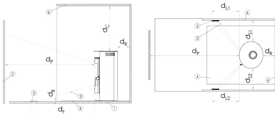
Abbildung 14 - Schematische Darstellung der Mindestabstände (siehe Tabelle 2)
