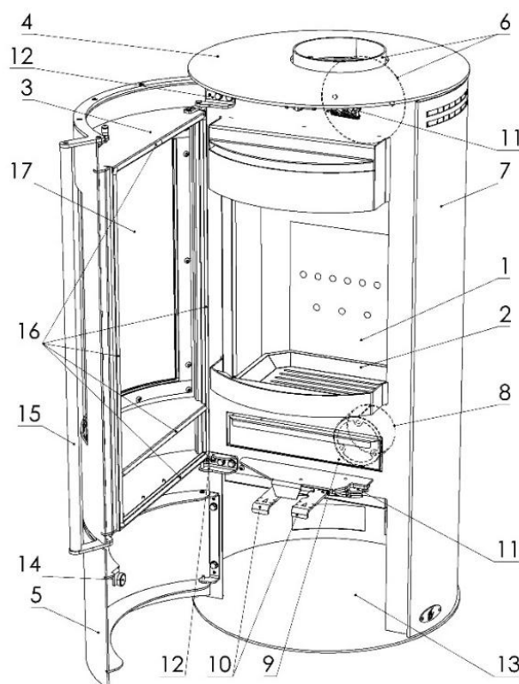
Abbildung 1 – Aufbau des Geräts
