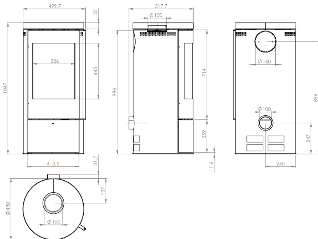
Abbildung 4 - Hauptmaße
