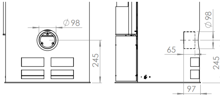
Abbildung 8- Verbrennungsluftanschluss
