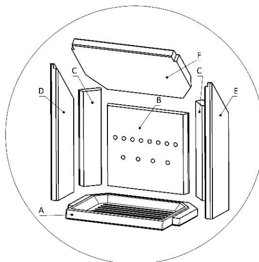
Abbildung 14 – Feuerraumauskleidung mit Rost
