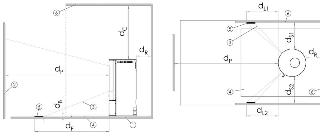
Abbildung 10 - Schematische Darstellung der Mindestabstände (siehe Tabelle 2)
