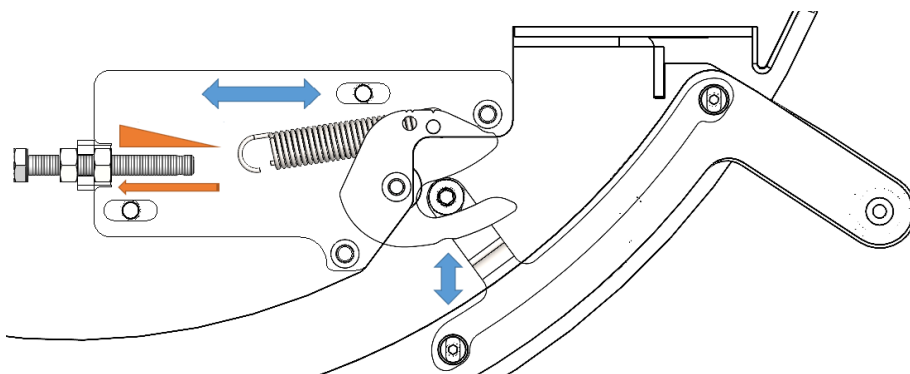
Abbildung 16 - Schnappverschluss
