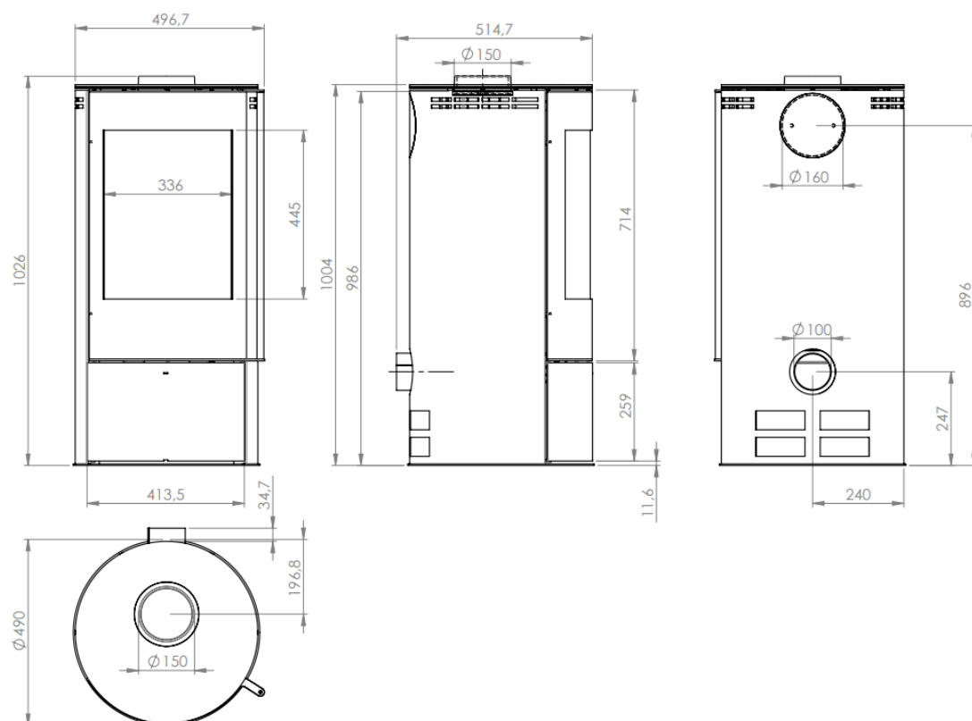
Abbildung 3 - Hauptmaße
