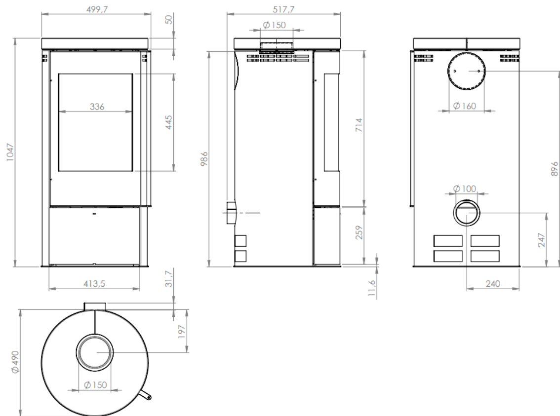
Abbildung 5 - Hauptmaße
