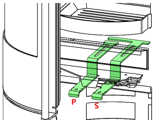
Abbildung 13 - P: Primärluftregler, S: Sekundärluftregler
