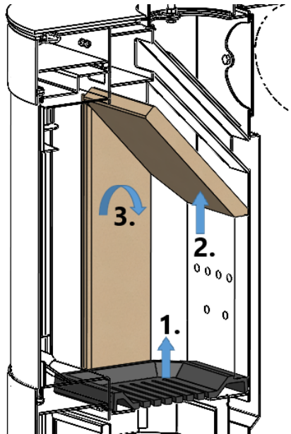
Abbildung 15 – Zugang zum Rauchraum
