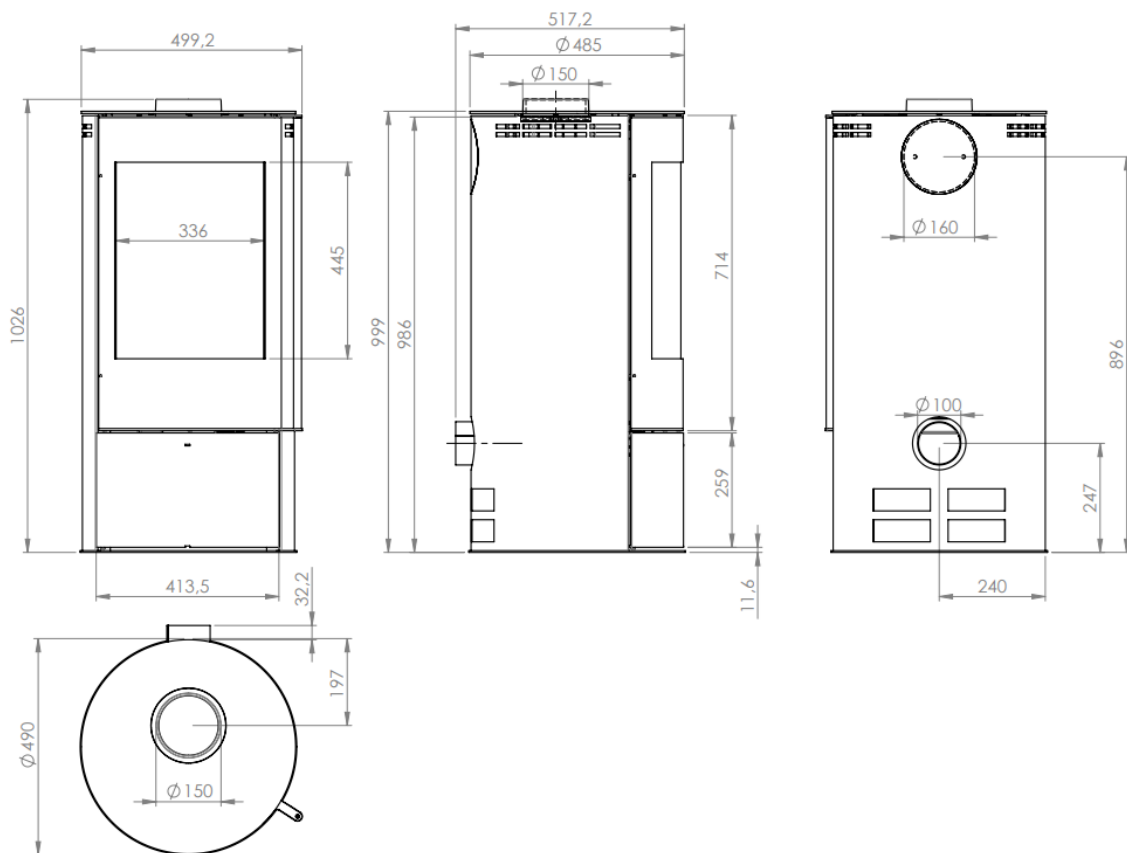
Abbildung 2 - Hauptmaße
