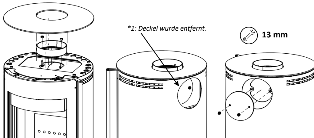
Abbildung 7 - Abgasstutzen und Abdeckung demontieren
