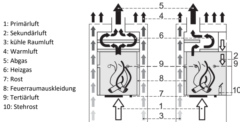
Abbildung 6 – Fire-Plus System, schematische Darstellung
