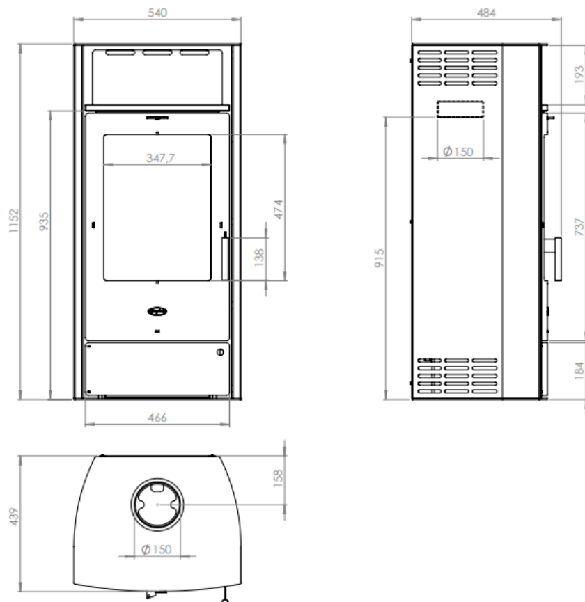
Abbildung 2 - Hauptmaße
