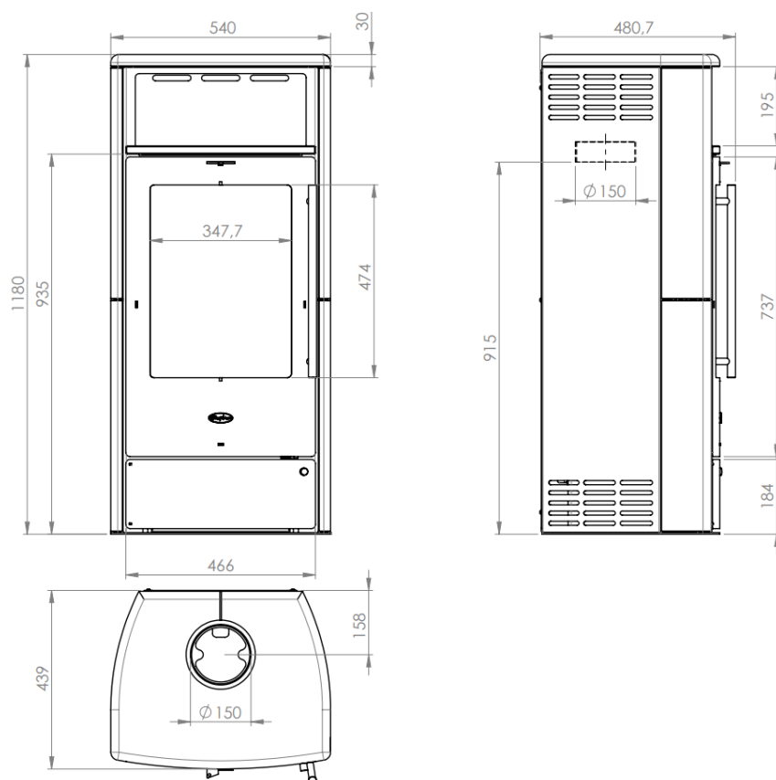
Abbildung 2 - Hauptmaße
