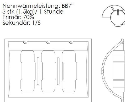
Abbildung 13 – Lufteinstellung und Brennstoffanordnung beim Betrieb mit Braunkohlenbriketts - Zeitbrandbetrieb
