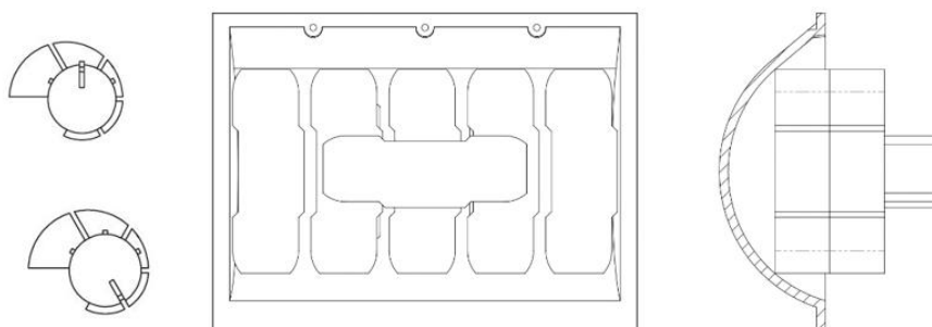
Abbildung 14 – Lufteinstellung und Brennstoffanordnung beim Betrieb mit Braunkohlenbriketts - Dauerbrandbetrieb
