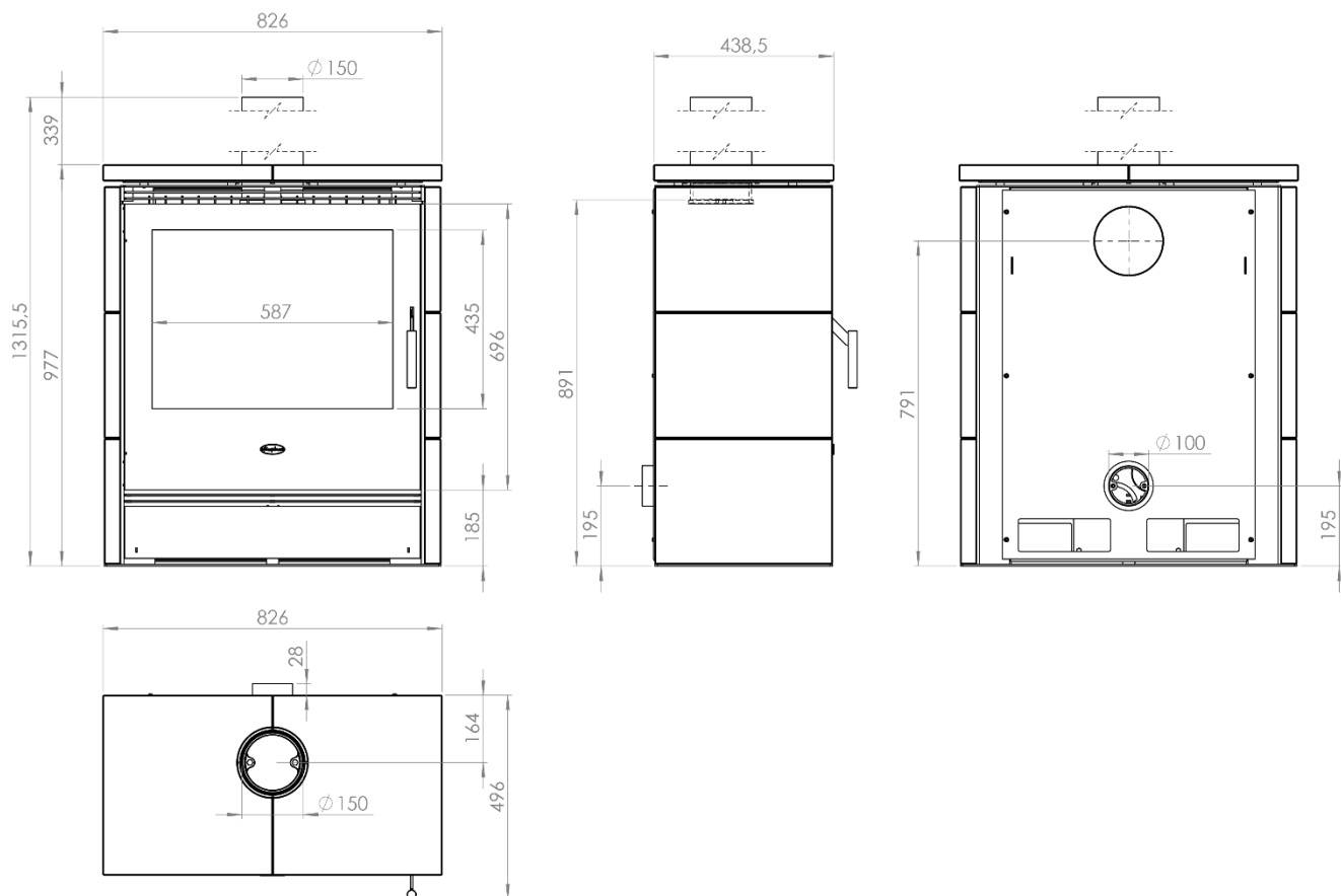
Abbildung 2 – Hauptmaße
