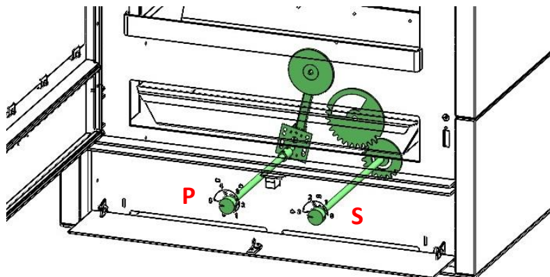
Abbildung 12 - Luftregelungsknöpfe
