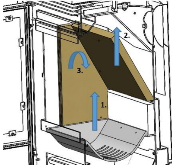
Abbildung 15 – Zugang zum Rauchraum
