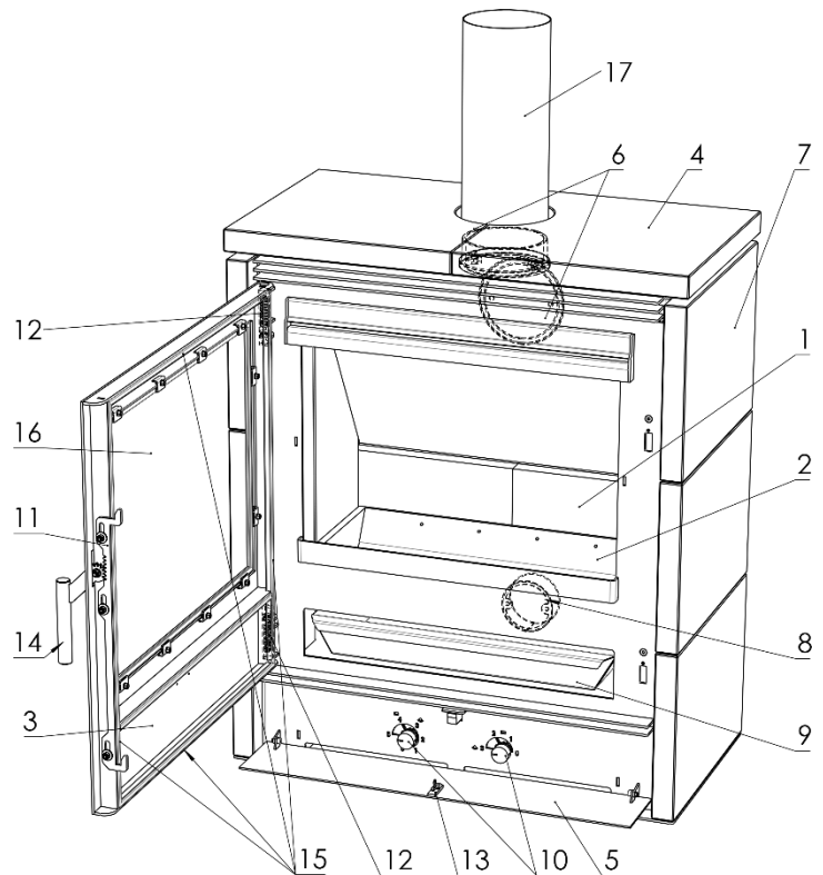
Abbildung 1 – Aufbau des Geräts
