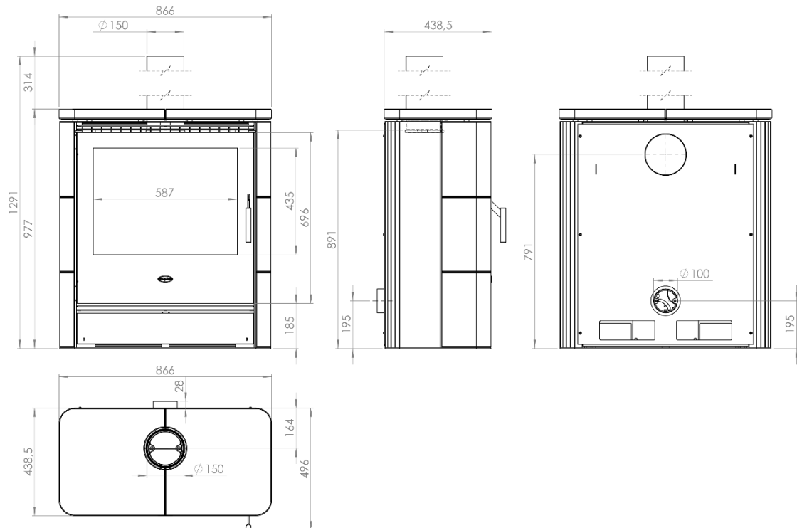
Abbildung 4 - Hauptmaße
