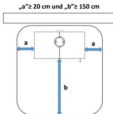
Abbildung 8 - Bodenplatte
