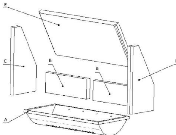
Abbildung 14 – Feuerraumauskleidung mit Rost
