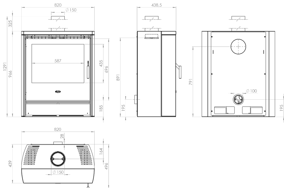
Abbildung 3 - Hauptmaße
