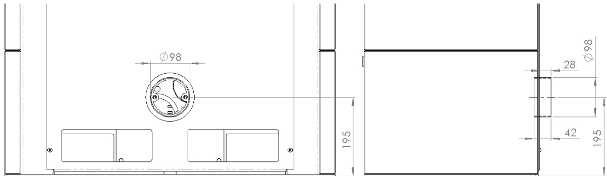
Abbildung 7- Verbrennungsluftanschluss
