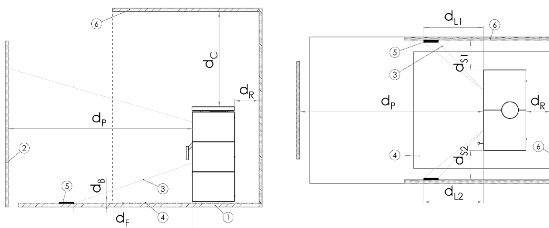
Abbildung 9 - Schematische Darstellung der Mindestabstände (siehe Tabelle 2)
