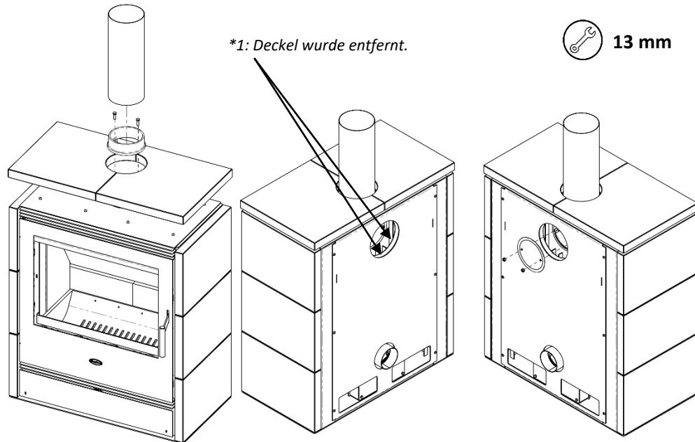
Abbildung 6 - Abgasstutzen und Abdeckung demontieren
