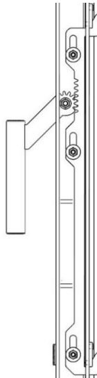
Abbildung 16 - Mehrfachverriegelung
