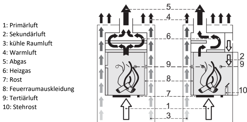
Abbildung 5 – Fire-Plus System, schematische Darstellung
