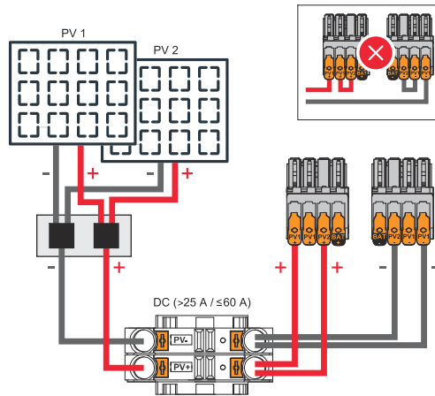
Kombinierte Solarmodul-Stränge mit Summenstrom größer 25 A ( I_{dcmax} ).
