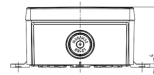
Mit Aussenbefestigungslasche/ with mounting lug
