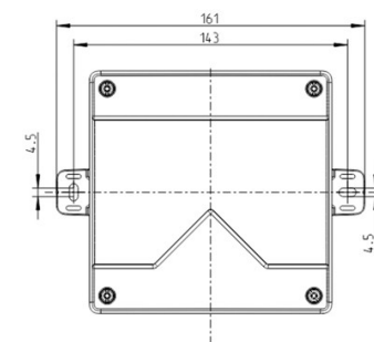
Mit Aussenbefestigungslasche/ with mounting lug
