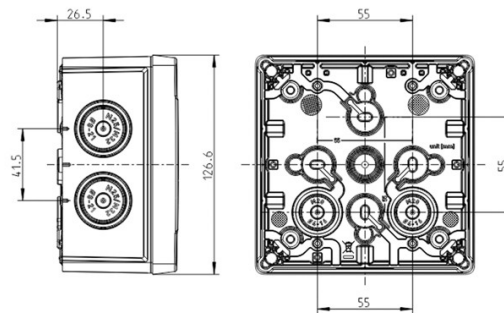
Isolierstopfen/insulating plug
