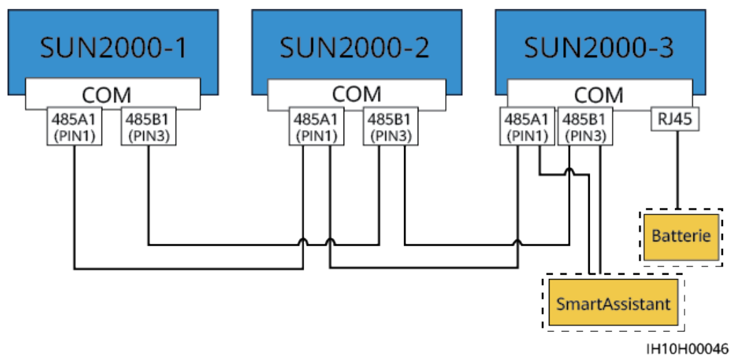
Abbildung 5-16 SmartAssistant-Vernetzung (die Komponente im gestrichelten Kasten ist optional)
