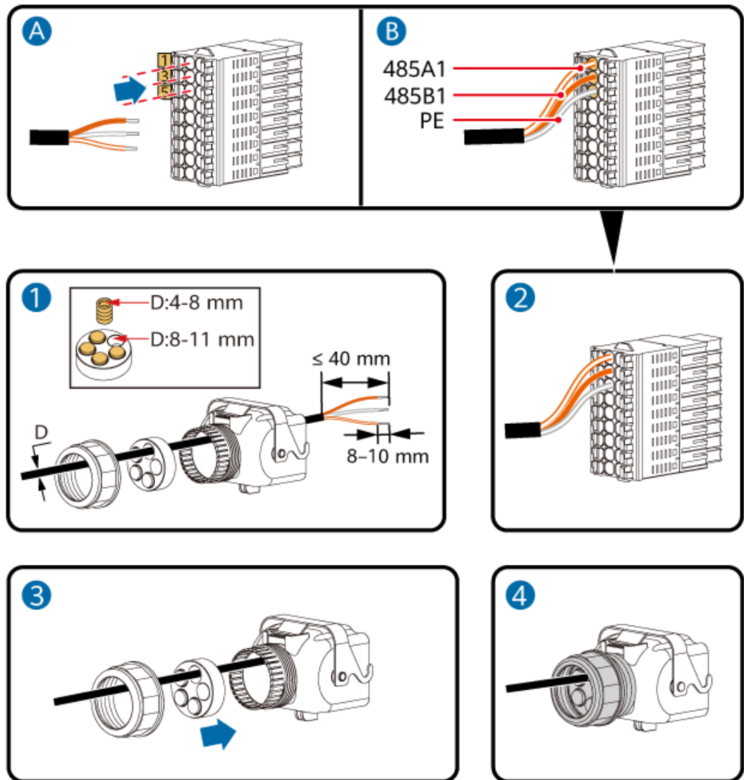
Abbildung 5-26 Kabelmontage
