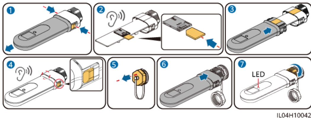
Abbildung 5-43 Installieren von 4G Smart Dongle (SDongleB-06)
