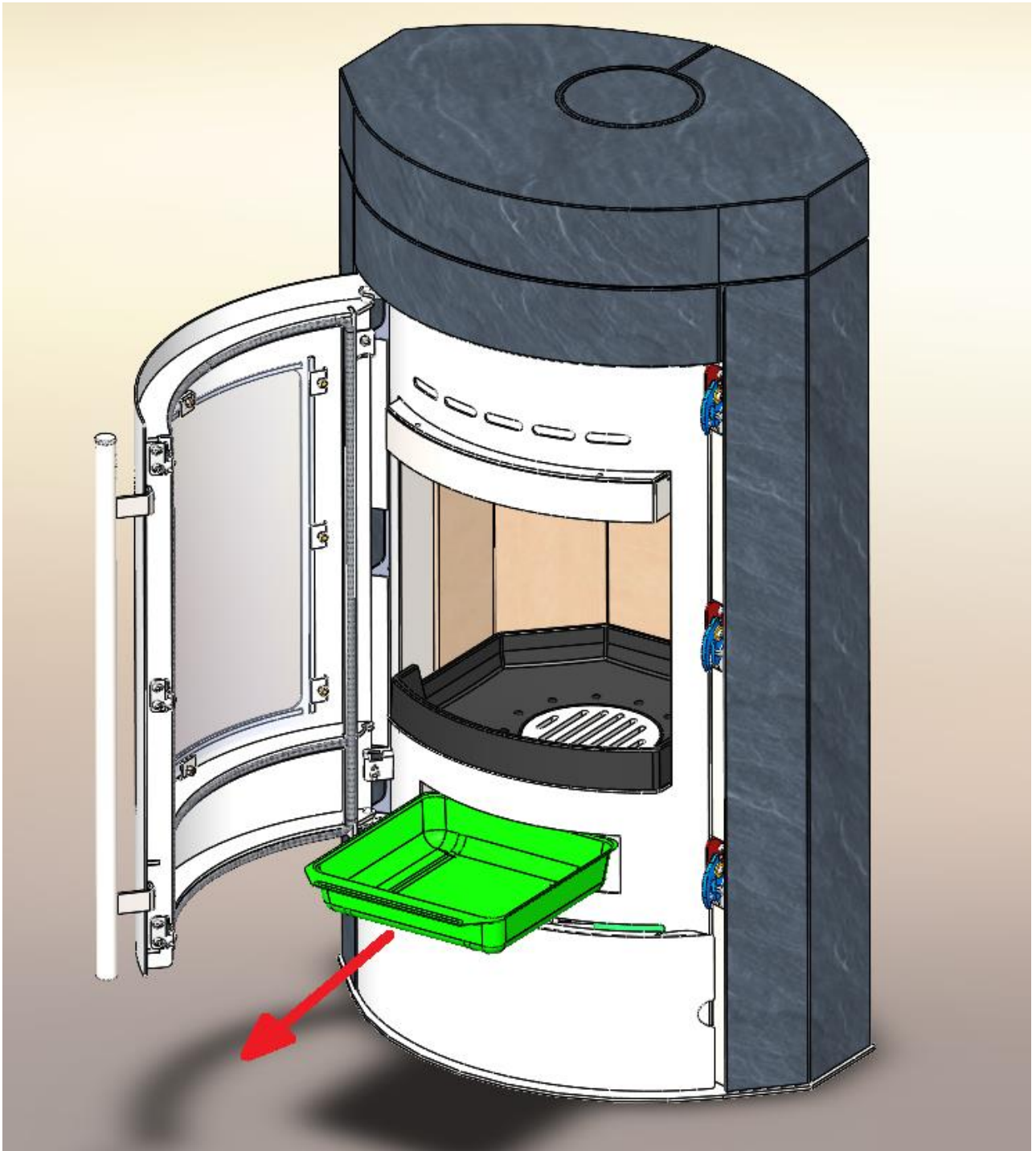
Abbildung 7 Entleeren der Aschelade
