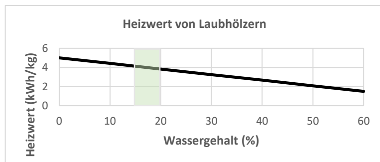
Abbildung 10 - Heizwertänderung in Abhängigkeit vom Wassergehalt
