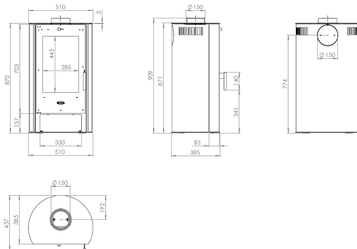
Abbildung 3 - Hauptmaße
