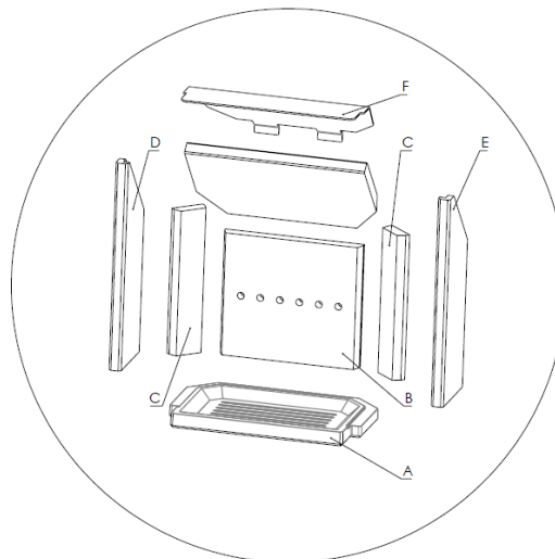
Abbildung 13 – Feuerraumauskleidung mit Rost
