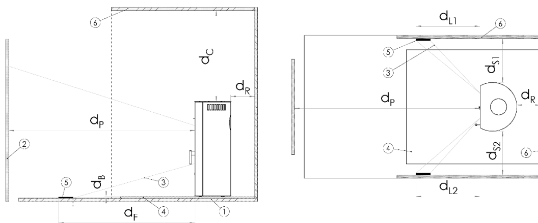
Abbildung 9 - Schematische Darstellung der Mindestabstände (siehe Tabelle 2)
