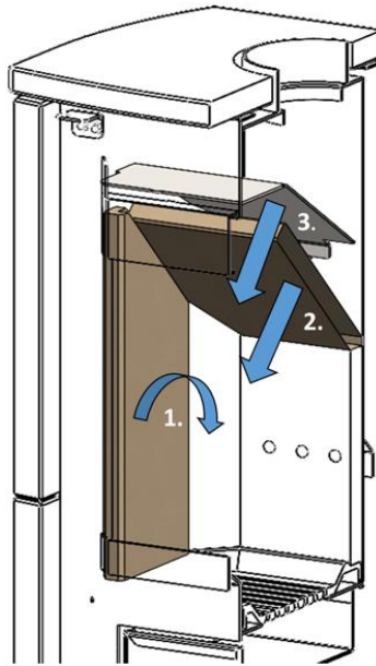
Abbildung 14 – Zugang zum Rauchraum
