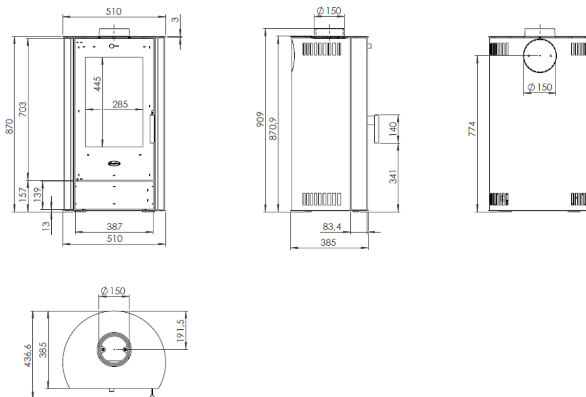
Abbildung 5 - Hauptmaße
