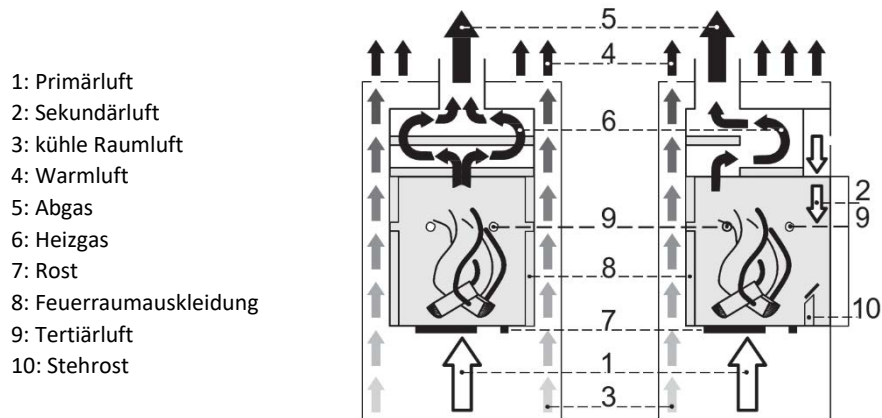
Abbildung 6 – Fire-Plus System, schematische Darstellung
