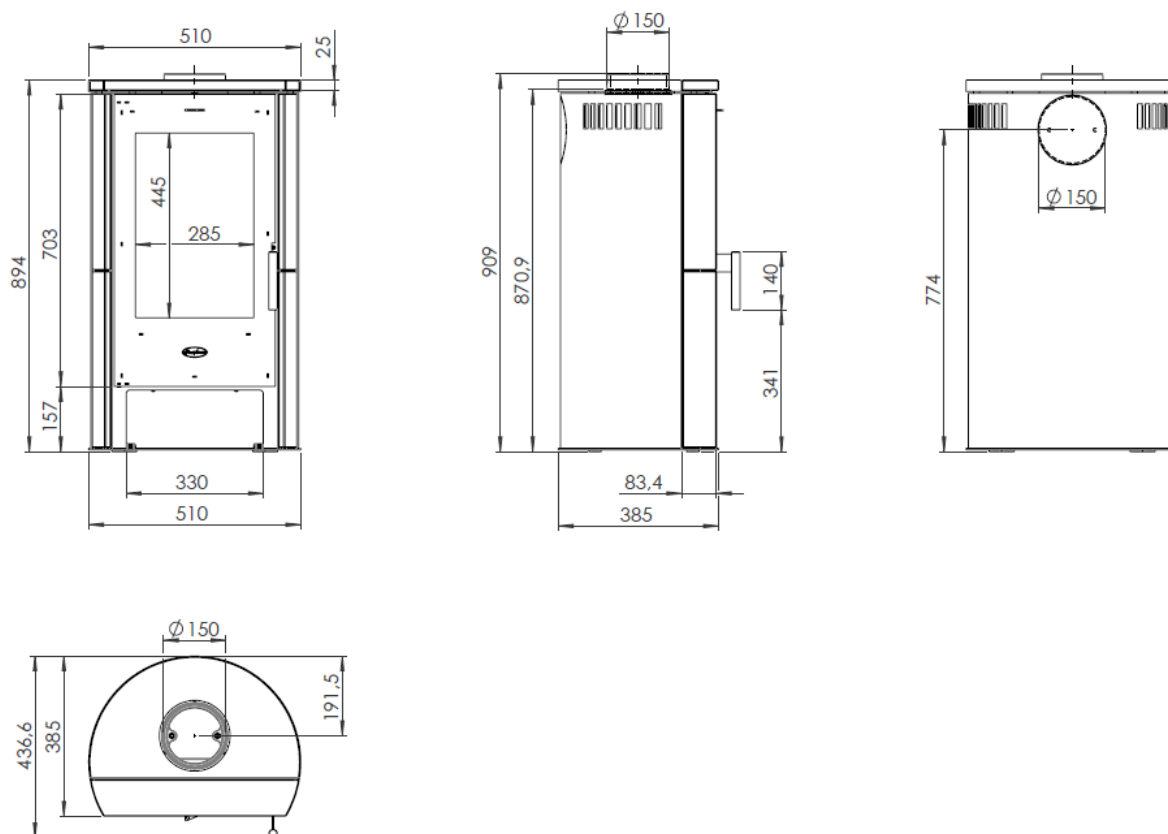
Abbildung 4 – Hauptmaße
