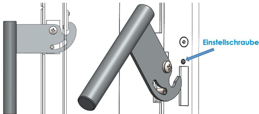
Abbildung 15 - Türverschluss
