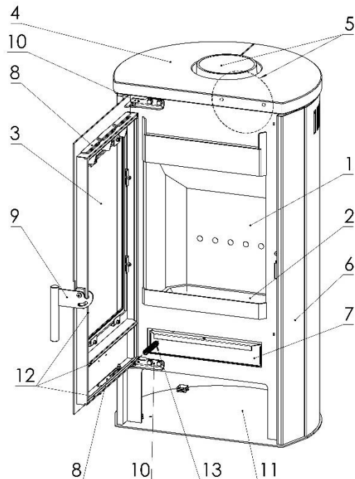
Abbildung 1 – Aufbau des Geräts
