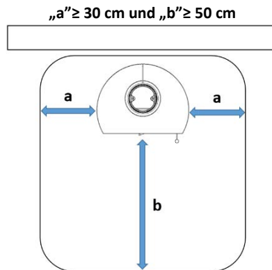
Abbildung 8 - Bodenplatte
