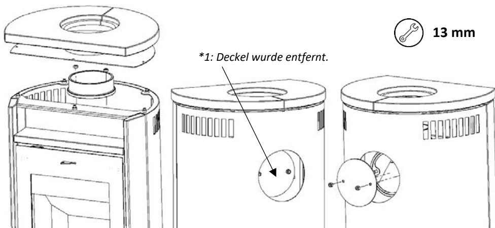
Abbildung 7 - Abgasstutzen und Abdeckung demontieren
