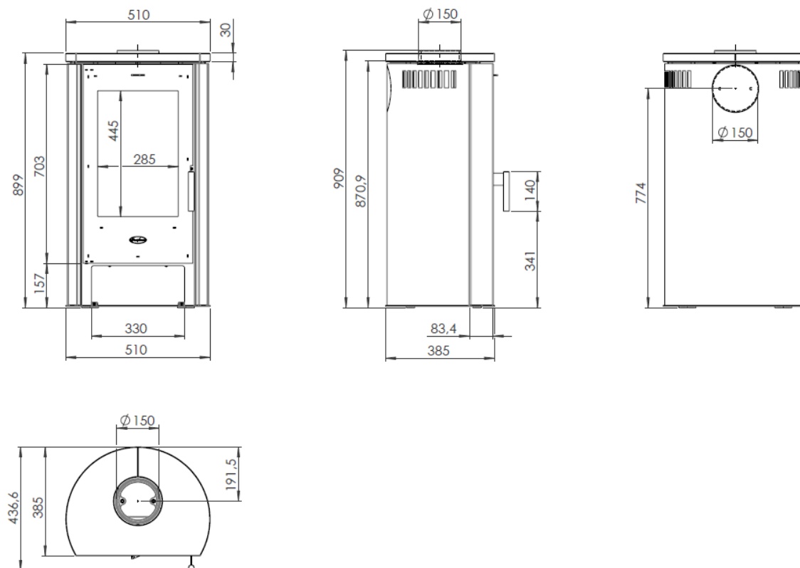
Abbildung 2 - Hauptmaße
