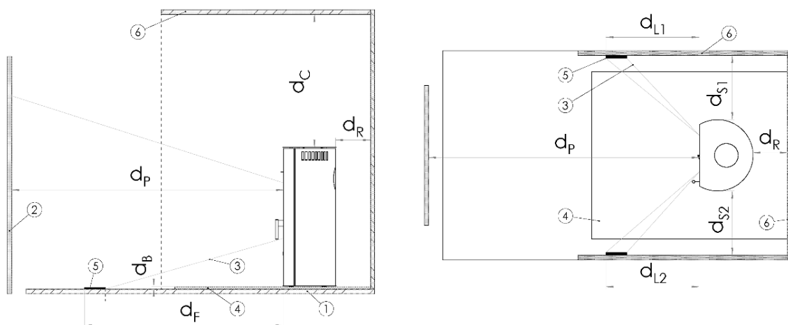
Abbildung 11 - Schematische Darstellung der Mindestabstände (siehe Tabelle 2)
