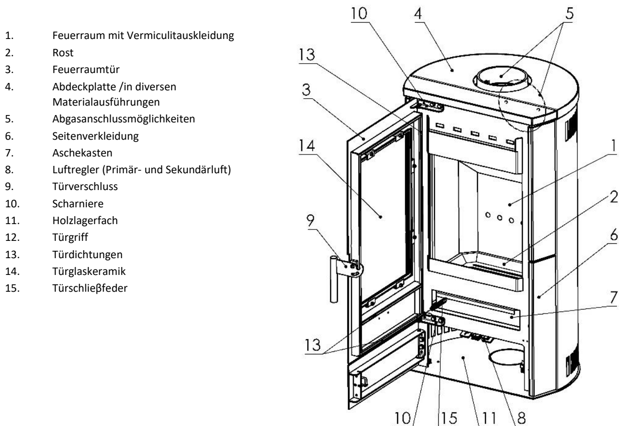
Abbildung 1 – Aufbau des Geräts
