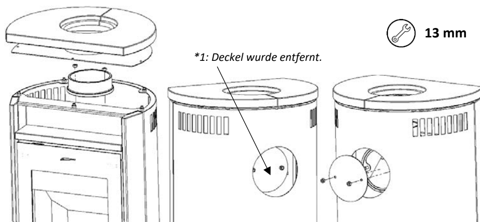
Abbildung 8 - Abgasstutzen und Abdeckung demontieren
