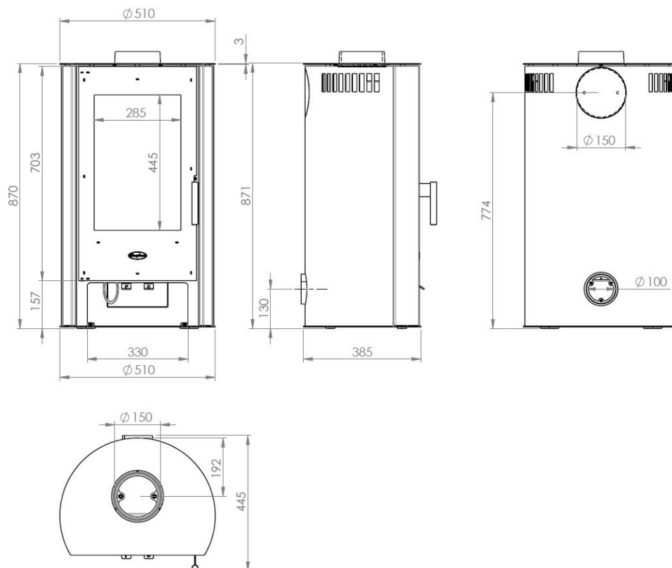
Abbildung 3 - Hauptmaße
