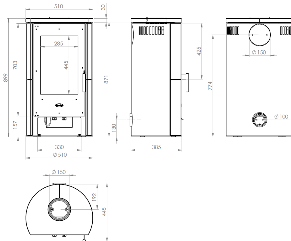
Abbildung 5 - Hauptmaße
