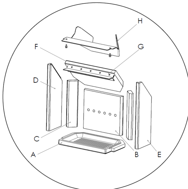
Abbildung 15 – Feuerraumauskleidung mit Rost
