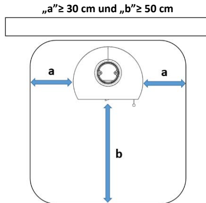
Abbildung 10 - Bodenplatte
