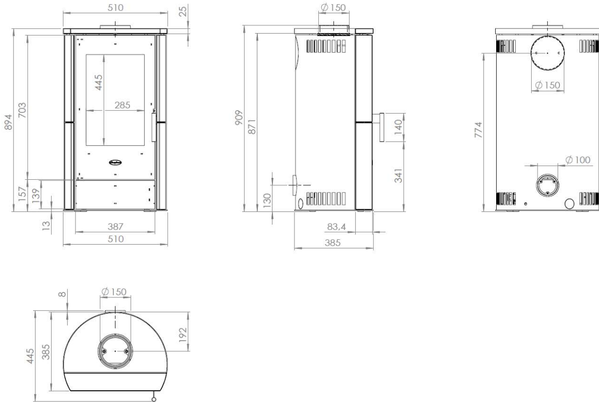
Abbildung 6 - Hauptmaße
