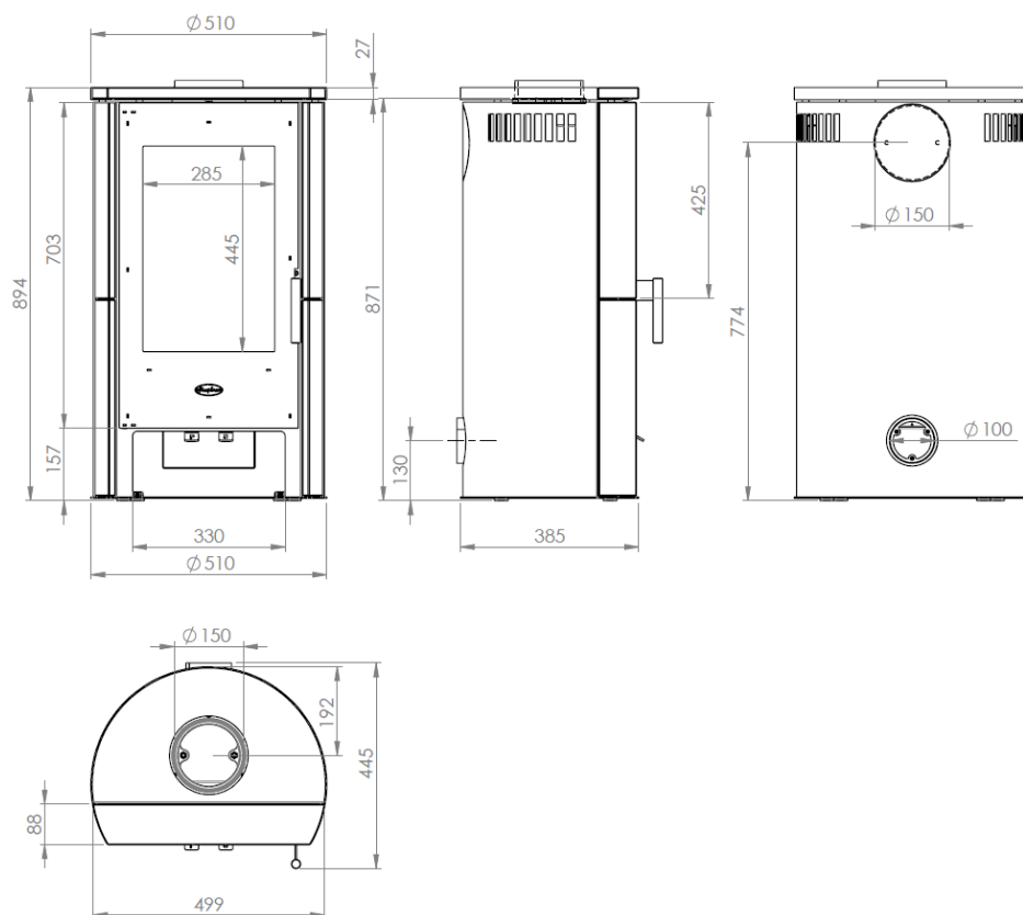
Abbildung 4 – Hauptmaße
