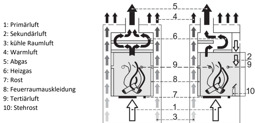
Abbildung 7 – Fire-Plus System, schematische Darstellung
