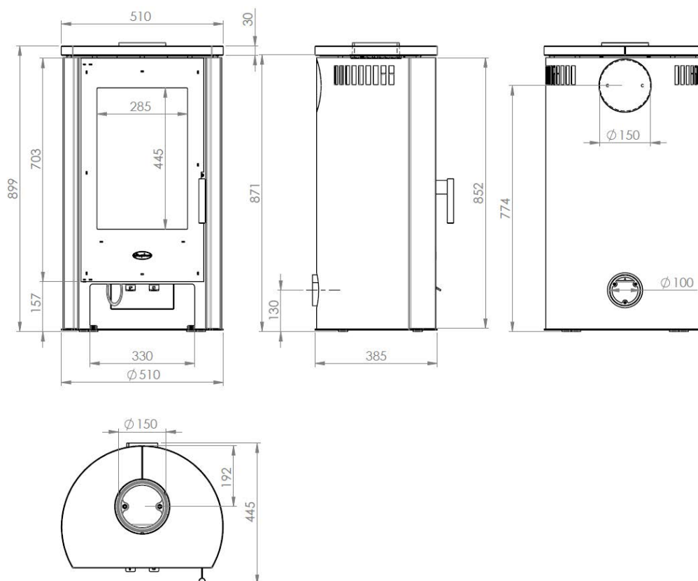
Abbildung 2 - Hauptmaße
