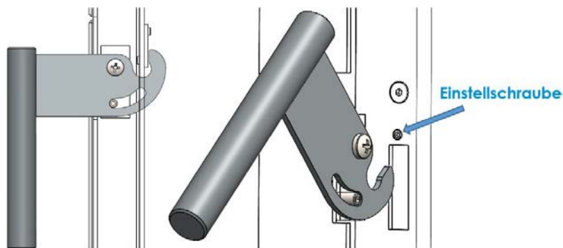
Abbildung 17 - Türverschluss
