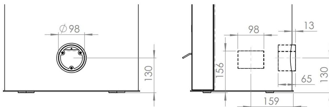
Abbildung 9 - Abgasstutzen und Abdeckung demontieren
