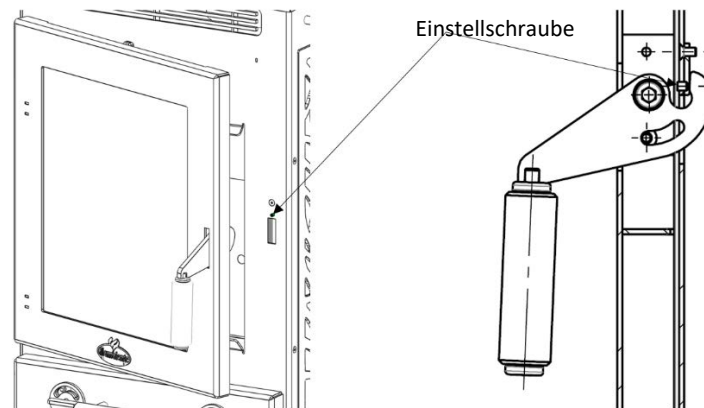
Abbildung 18 – Türschloss
