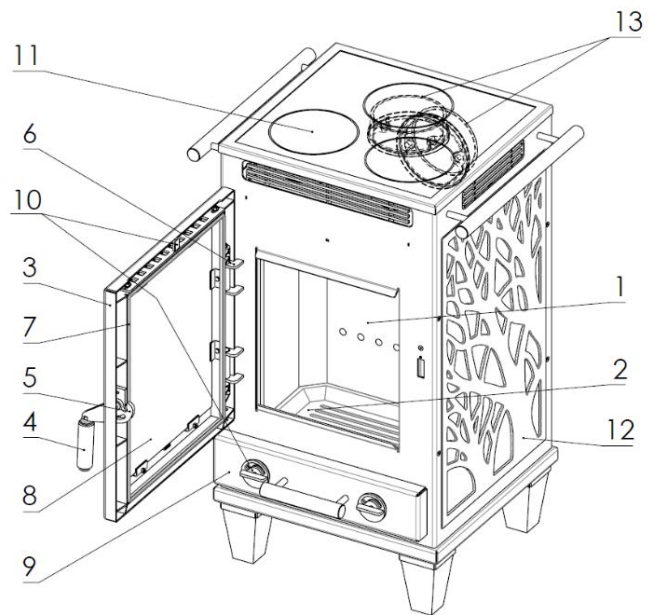
Abbildung 2 – Aufbau des Geräts
