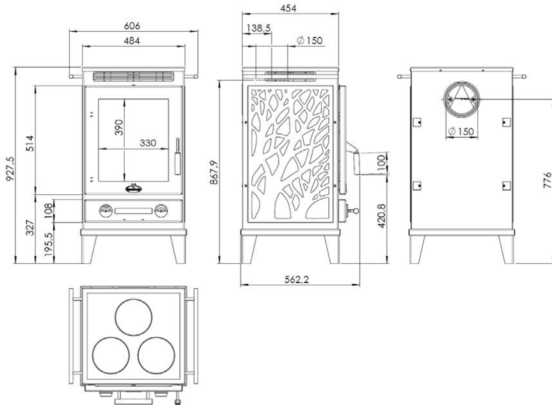
Abbildung 5 – Hauptmaße
