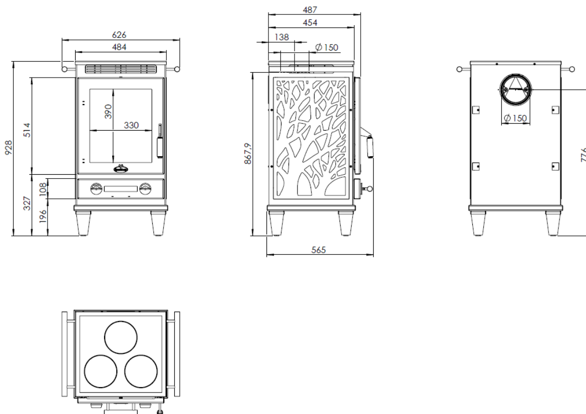
Abbildung 4 – Hauptmaße
