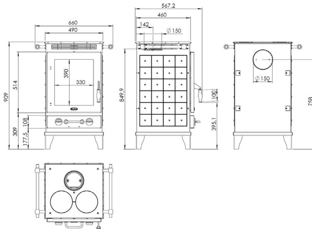
Abbildung 3 – Hauptmaße
