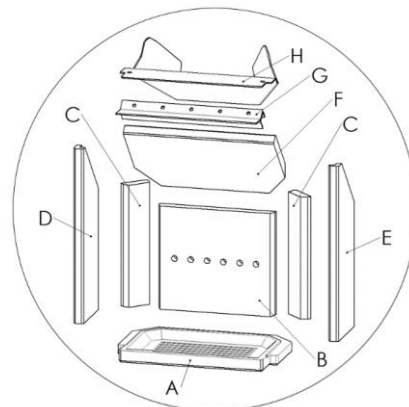
Abbildung 16 – Feuerraumauskleidung mit Rost
