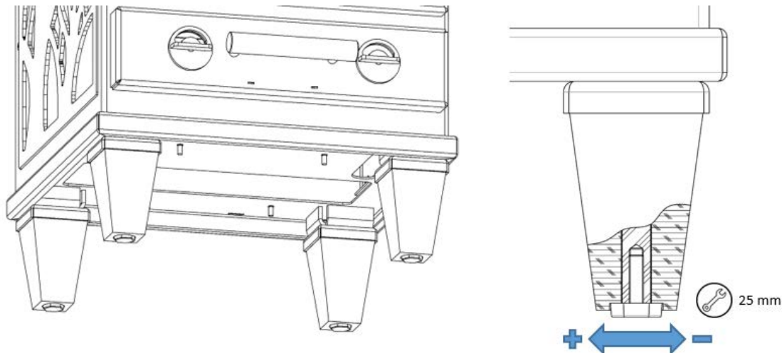
Abbildung 9 – Höhenverstellbare Füße
