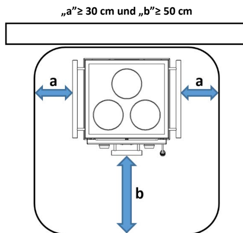
Abbildung 10 – Bodenplatte
