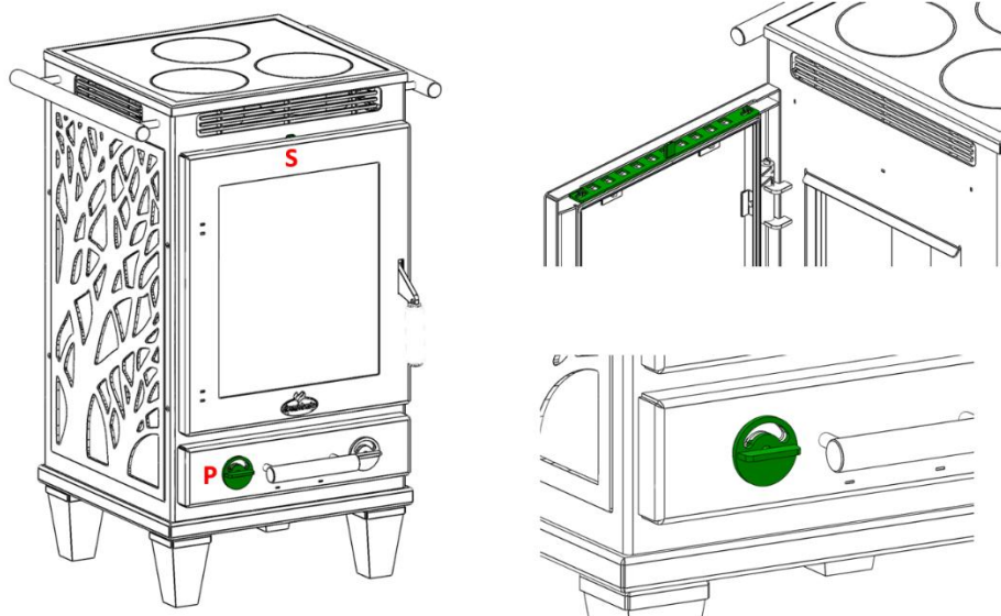
Abbildung 14 – P: Primärluftregler, S: Sekundärluftregler
