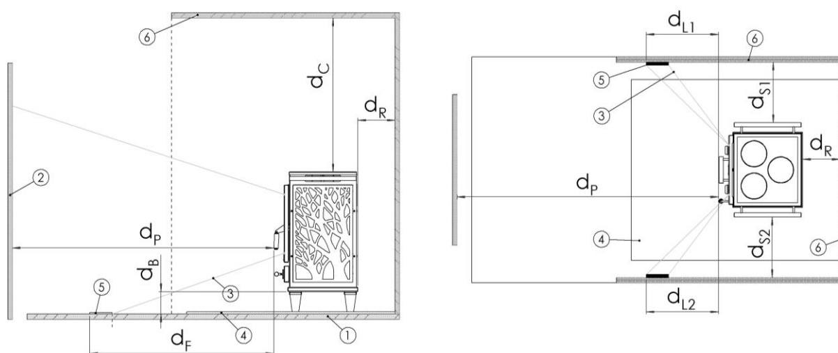
Abbildung 11 – Schematische Darstellung der Mindestabstände (siehe Tabelle 2)
