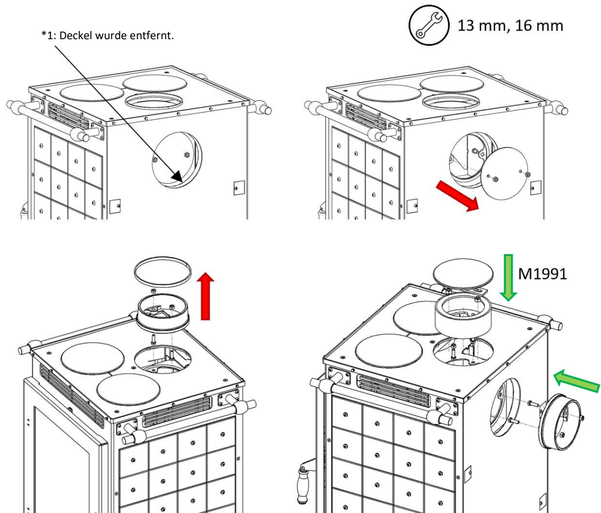
Abbildung 7 – Umrüstung auf hinteren Anschluss – K7250 + M1991
