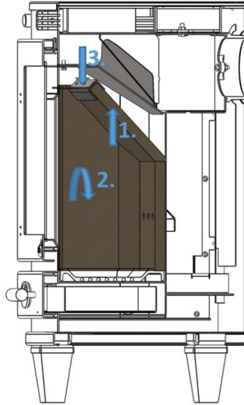
Abbildung 17 – Zugang zum Rauchraum
