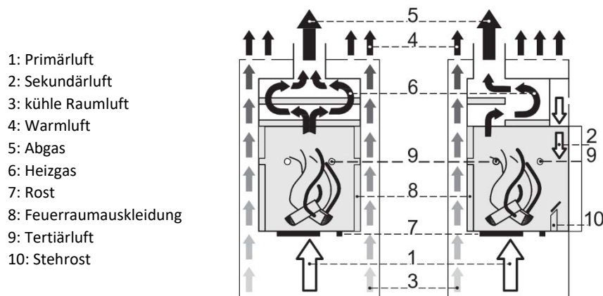
Abbildung 6 – Fire Plus System, schematische Darstellung
