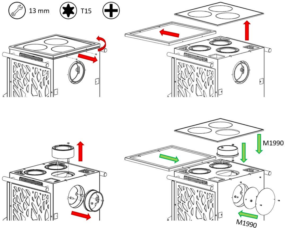
Abbildung 8 – Umrüstung auf oberen Anschluss – K7251/K7252 + M1990
