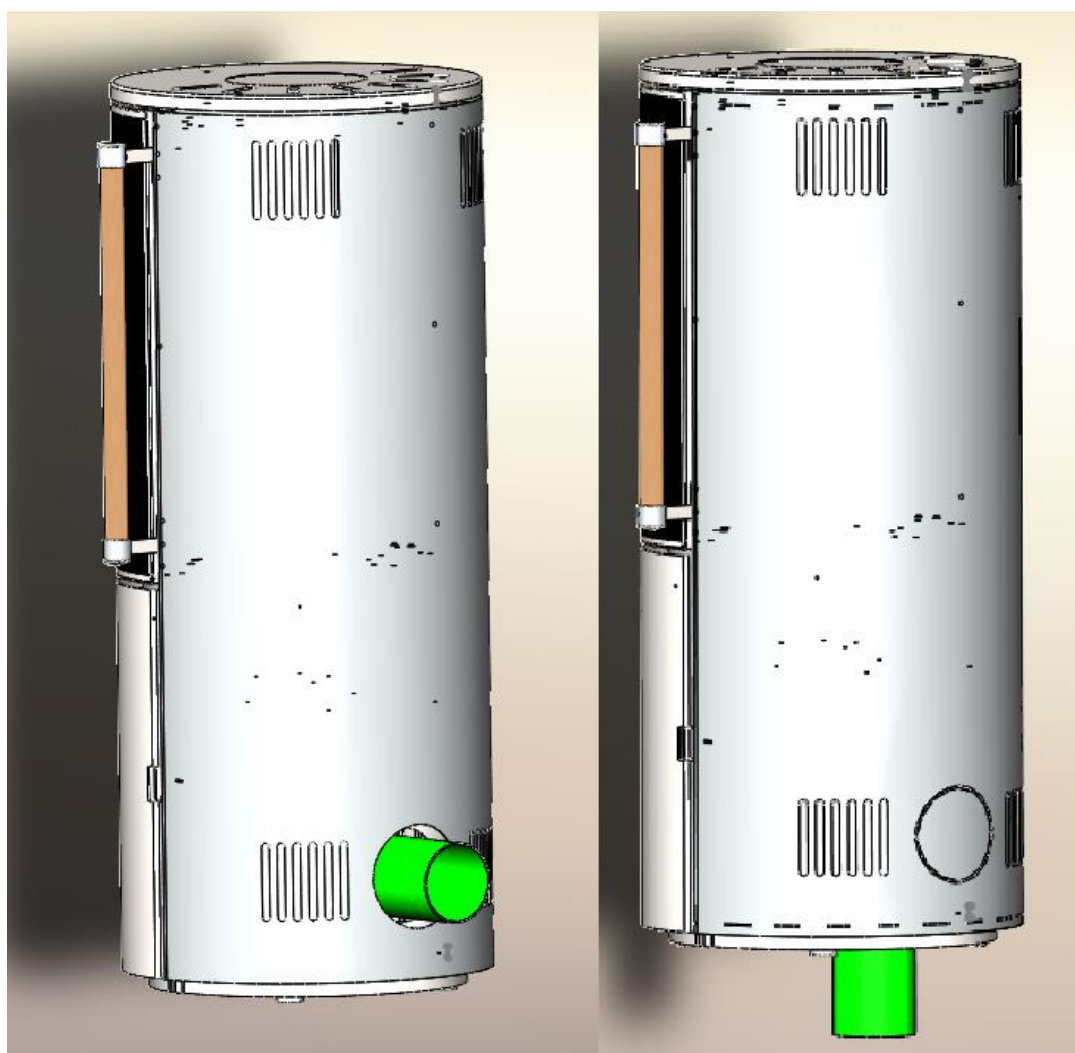
Figura 4 Racord pentru aer exterior în spate / în partea de jos
