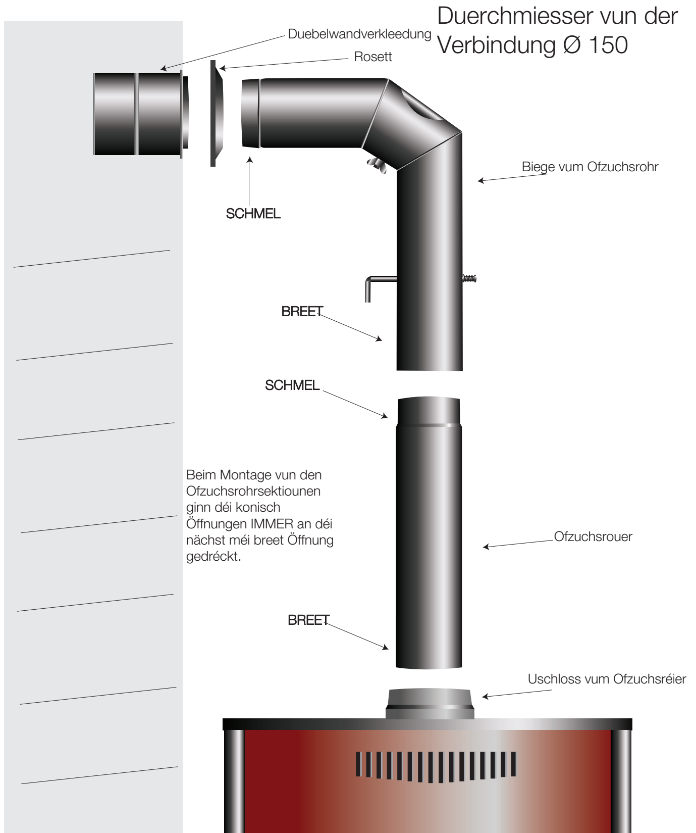
Figur 5 Uschloss vum Holzuewen un de Kamäin
