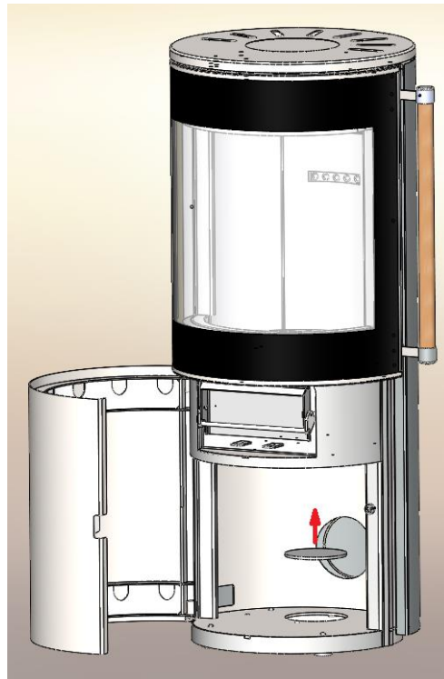
Figur 3 Mikrospalt fir d'Loftzoufuhr vun dobaussen um Réck / ënnen schneiden
