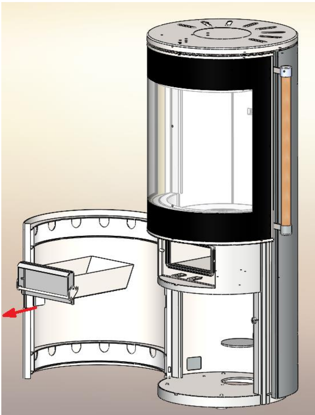
Figure 7 Vider le tiroir à cendres
