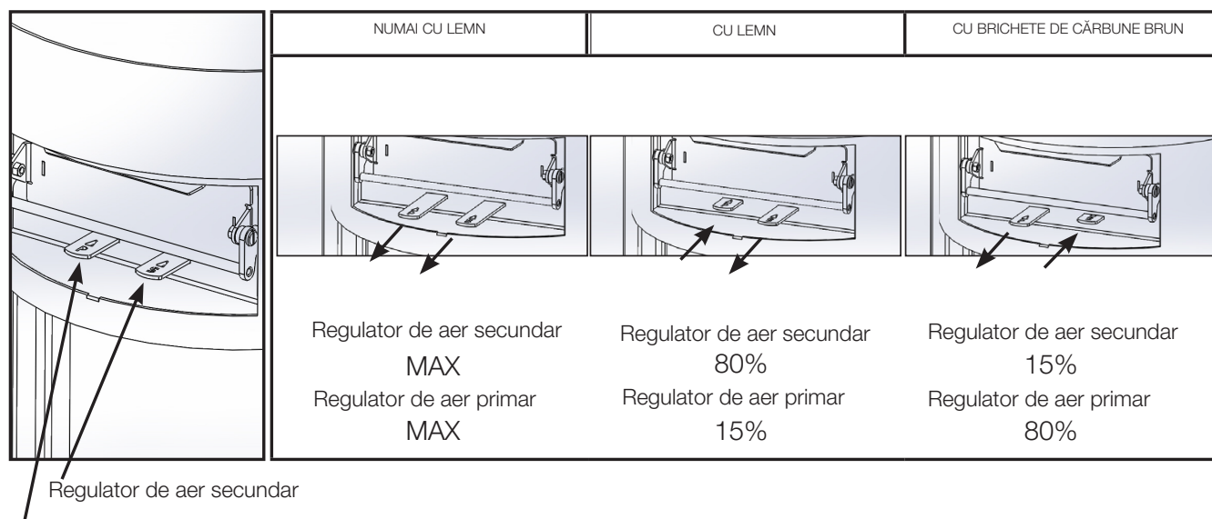
Figura 6 Utilizarea regulatorului de aer
