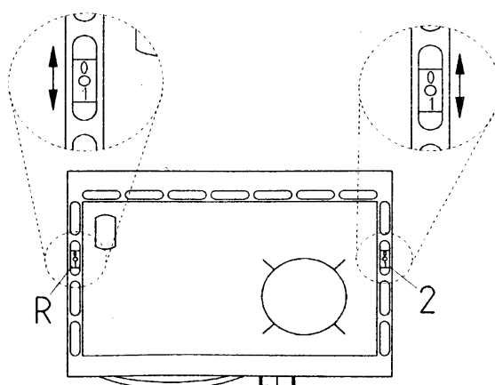
Ansicht: Rauchabzug links Bei Rauchabzug rechts spiegelverkehrt
