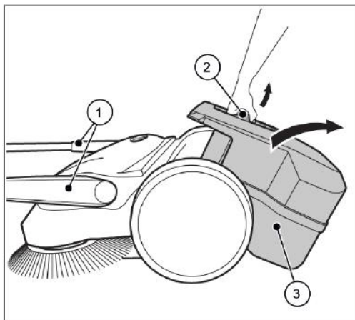
Fig. 11: Tøm oppsamler
