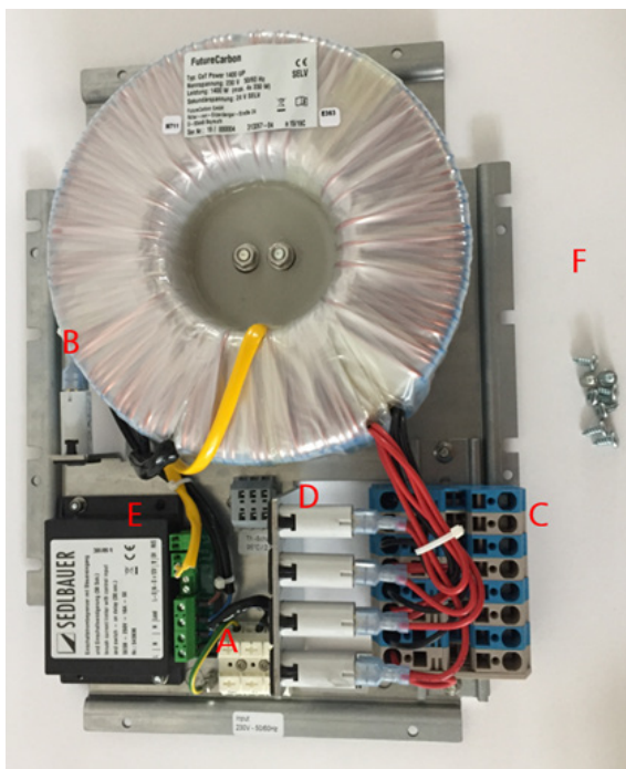
Abbildung 1: Übersicht der Spannungsversorgung und deren Komponenten
