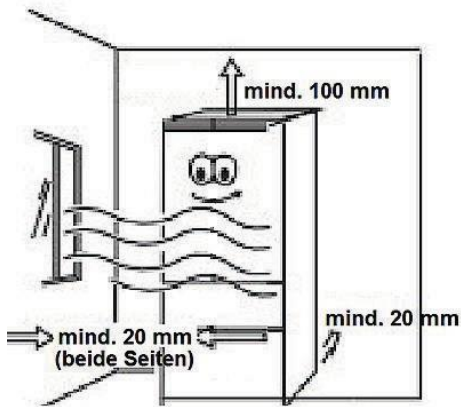
RAUMBEDARF DES GERÄTES INKL. DER MINDESTABSTÄNDE FÜR EINE ORDNUNGSGEMÄßE BELÜFTUNG BEI GESCHLOSSENEN TÜREN
