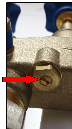
Śruba z rowkiem do regulacji twardości
