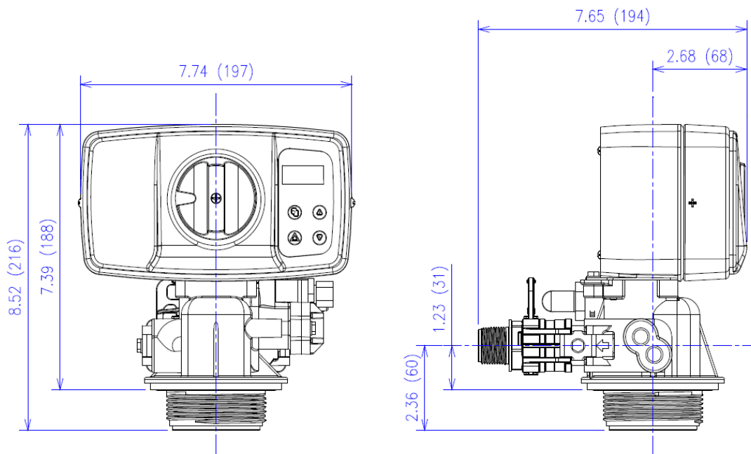
Rozměry regulačního ventilu
