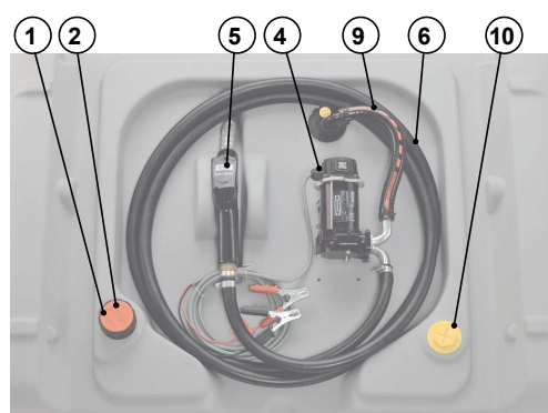
DT-Mobil Easy 440 I cu pompă 12V 40 l/min
