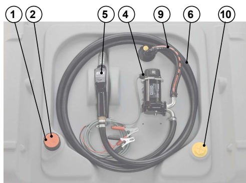
DT-Mobil Easy 440I pumpulla 12 V 40 l/min
