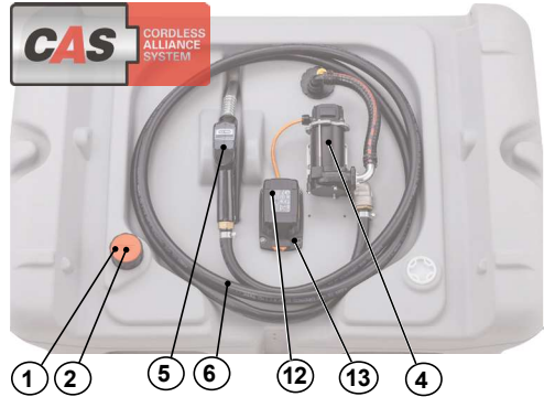
Vista interna DT-MOBIL Easy 440 I
