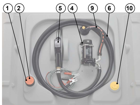
DT-Mobil Easy 440I med pump 12V 40 l/min
