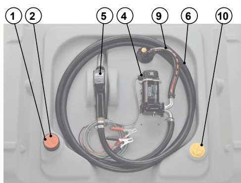
DT-Mobil Easy 440 I z pompą 12 V 40 l/min
