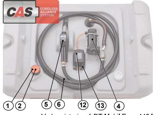
Vedere interioară DT-Mobil Easy 440 I
