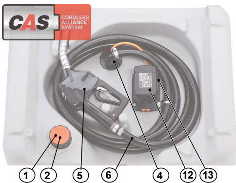
Innenansicht DT-Mobil Easy 210 I
