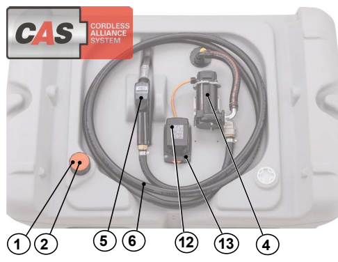
Innenansicht DT-Mobil Easy 440 I
