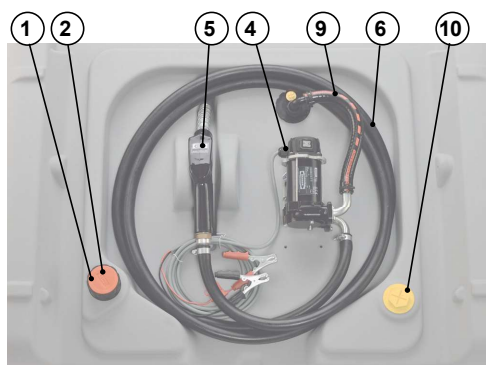
DT-Mobil Easy 440 I met pomp 12 V 40 l/min.
