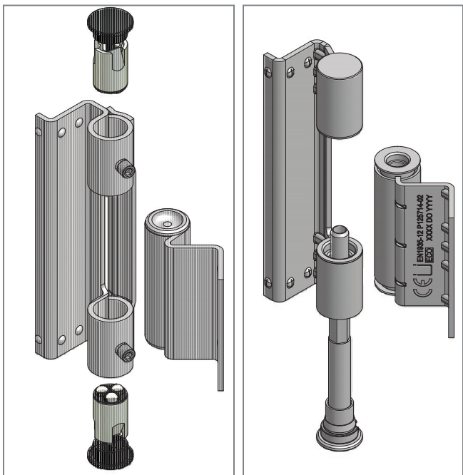
Bandsystem Variante 1
