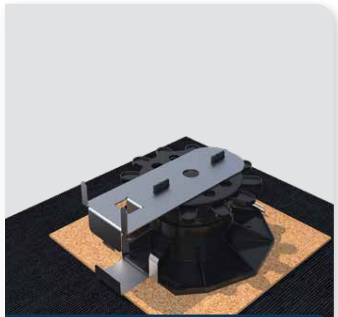
Ober- und Unterprofil an den Verstellfuß anbringen
