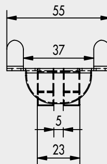
Vorderansicht
