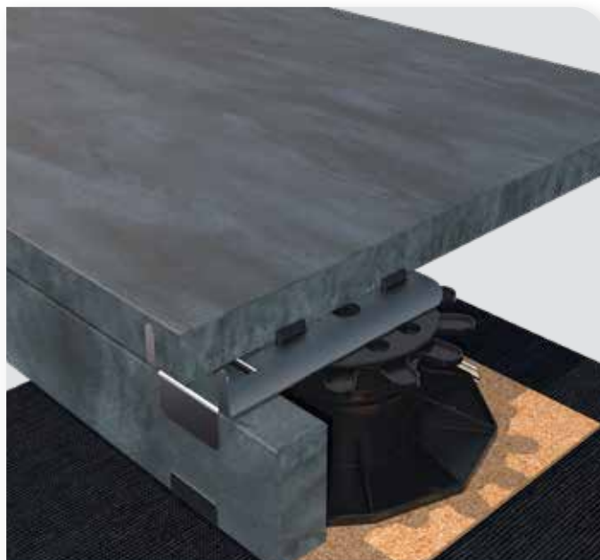
Randstein in die Führung des Systemc Stedgefix schieben
