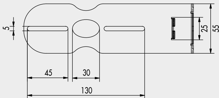
Draufsicht
