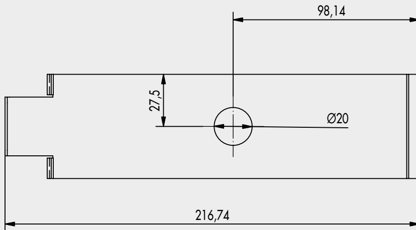
Draufsicht
