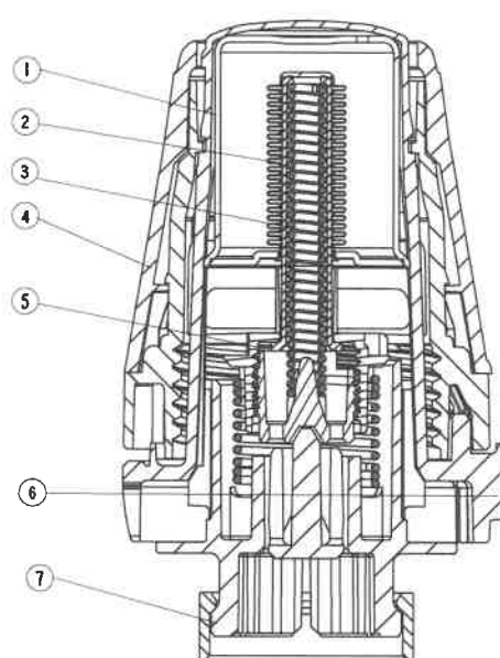
Danfoss Regus® M30
