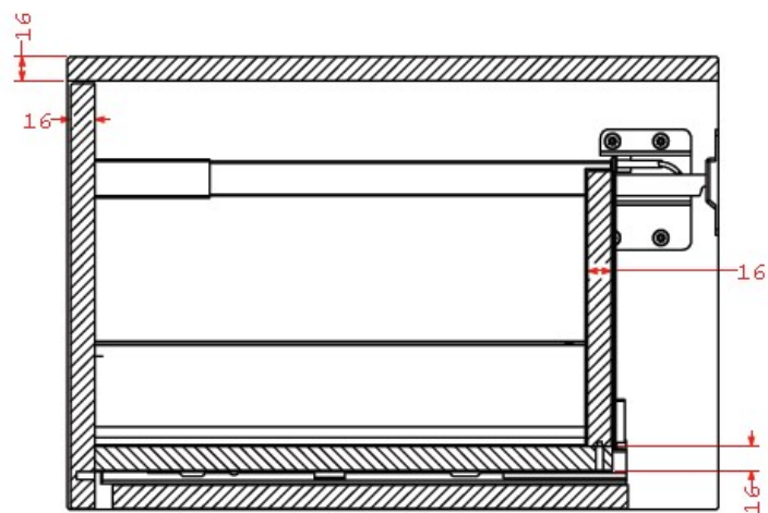
SEZIONE B-B SCALA 1 : 5
